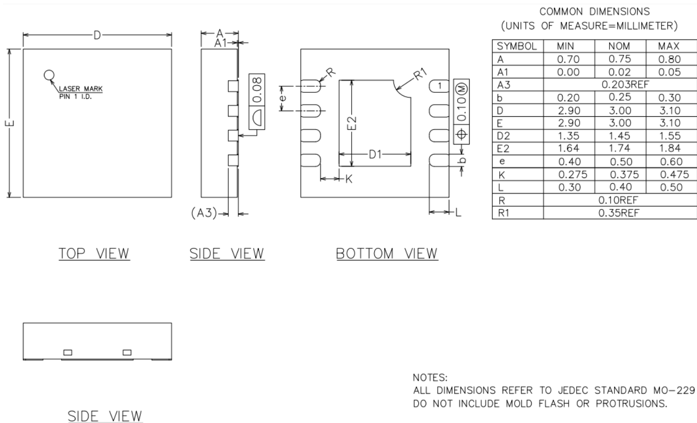
图 31. DFN-8 封装 (3mmx3mm)
