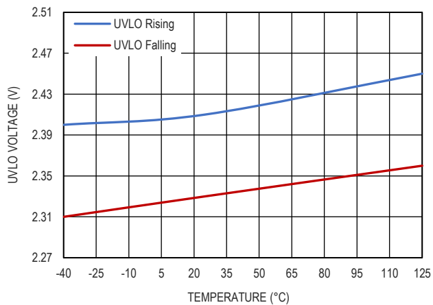
图 17. UVLO 阈值
