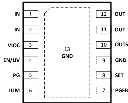
图 6. GM12051ACPZ-1 引脚配置(顶视图)
