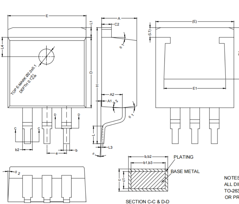
图 21.3 引脚 TO-263
