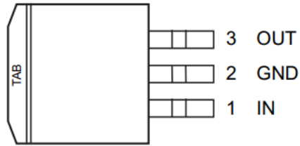
3 引脚 TO-263 裸露焊盘必须焊接到 PCB 上
