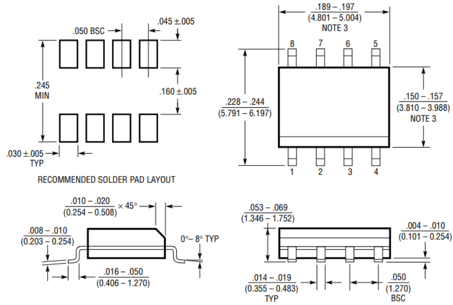
图 29.8 引脚 SO-8
