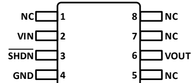
图 1. 8 引脚 MSOP
