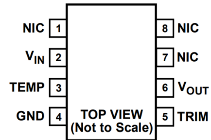
图 2. 8 引脚 SOIC
