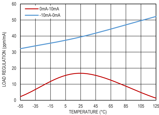
图 9. 负载调整率和温度的关系, V_{OUT}=1.25V
