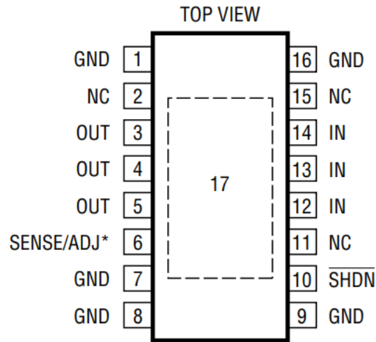
16 引脚 TSSOP
