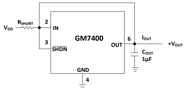
图 27. 正压并联方式
