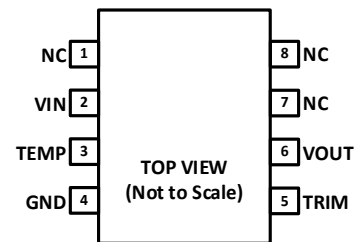
图 2. 8 引脚 SOIC
