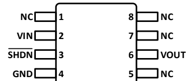
图 1. 8 引脚 MSOP
