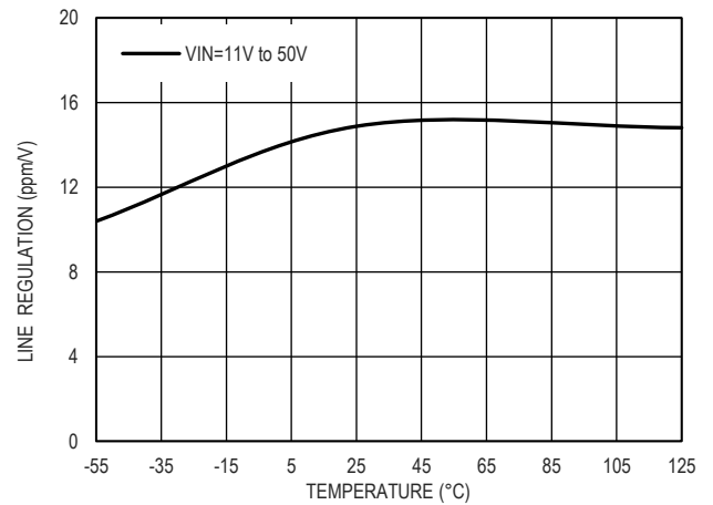
图 17. 输入调整率和温度的关系, V OUT =4.096V
