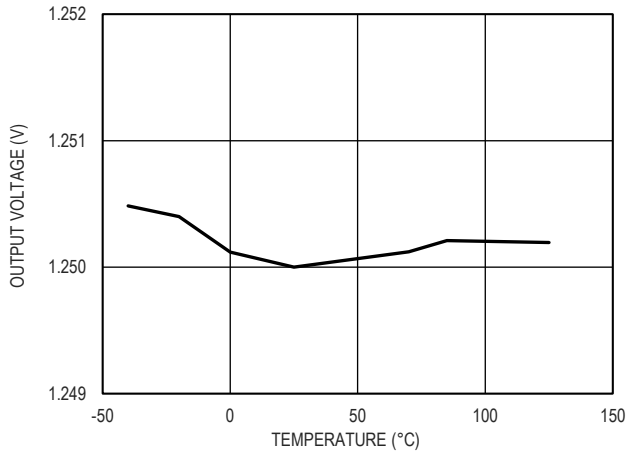
图 6. 1.25V 输出电压和温度的关系
