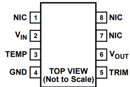
图 2. 8 引脚 SOIC
