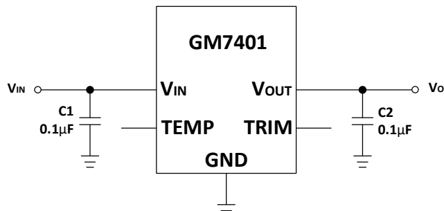
图 26. 有电容的应用电路
