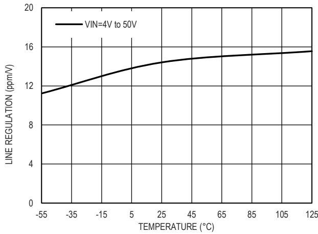
图 14. 输入调整率和温度的关系, V OUT =1.25V
