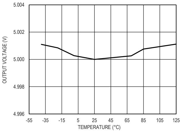
图 8. 3.3V 输出电压和温度的关系
