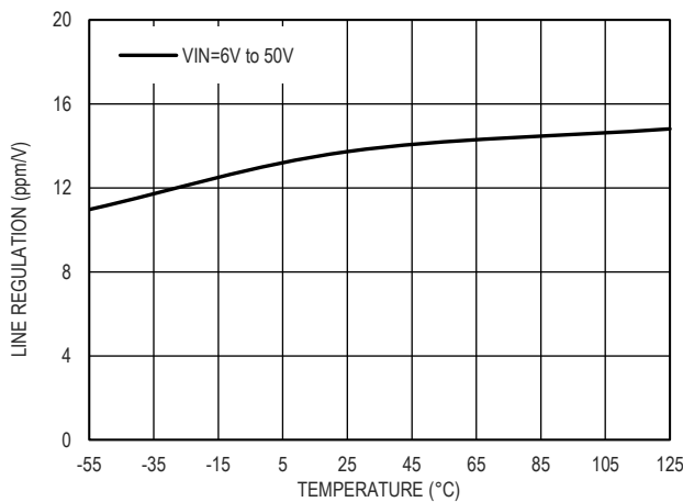
图 16. 输入调整率和温度的关系, V OUT =3.3V
