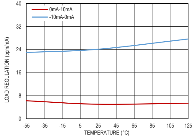
图 13. 负载调整率和温度的关系, V OUT =4.096V
