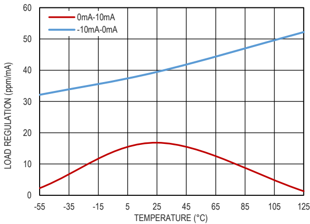
图 10. 负载调整率和温度的关系, V_{OUT}=1.25V
