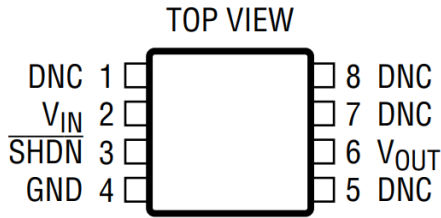
图 3. MSOP-8 引脚配置(顶视图, GM7400)
