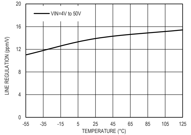
图 15. 输入调整率和温度的关系, V OUT =2.048V
