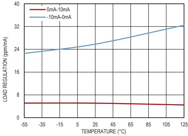
图 12. 负载调整率和温度的关系, V OUT =3.3V
