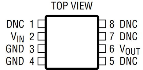
图 4. MSOP-8 引脚配置(顶视图, GM7400-1)
