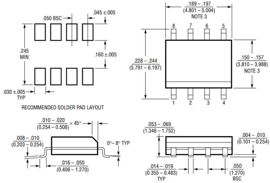
图 30.8 引脚 SO-8
