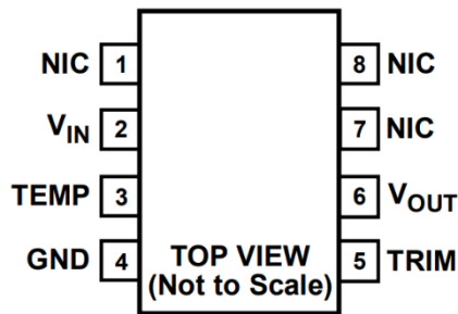
图 5. SO-8 引脚配置(顶视图)
