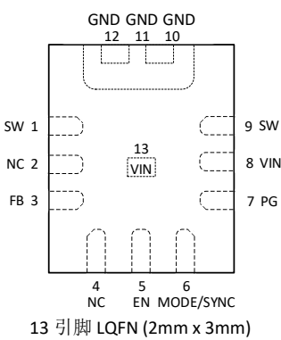
图 5 引脚配置
