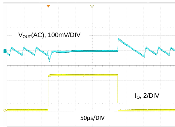
图 25. V_{OUT} = 1.2V , I_O = 0.1A 至 4.5A , 低功耗模式
