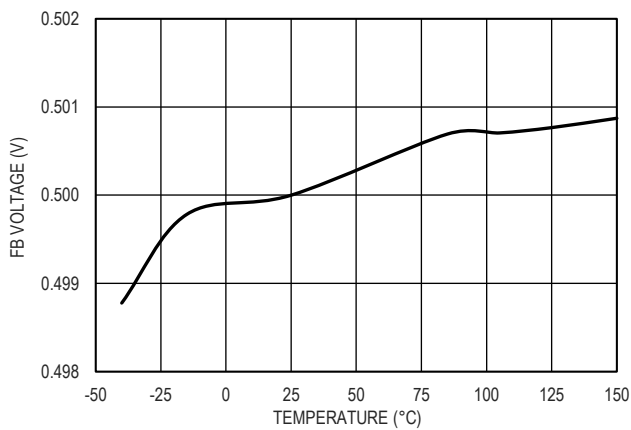
图 10. FB 引脚电压和温度的关系
