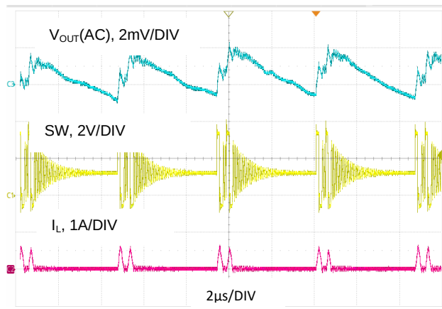
图 21. V_{OUT} = 1.2V , I_O = 100mA , PSM 模式
