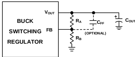
图 26. 反馈电阻网络
