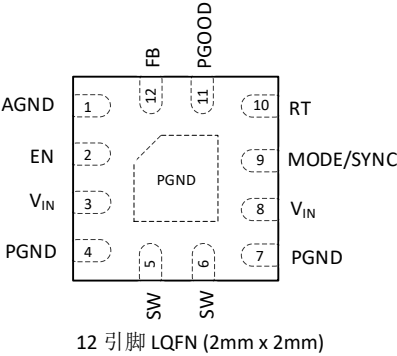
图 4 引脚配置
