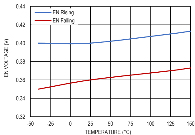
图 16. EN 阈值和温度的关系
