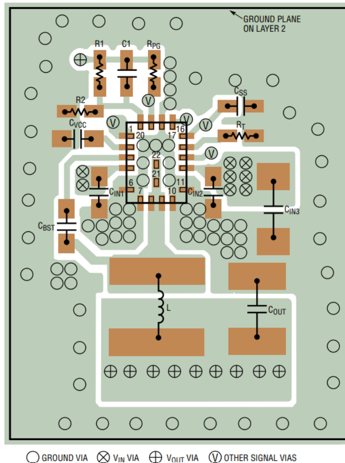
图 5. PCB 布局推荐
