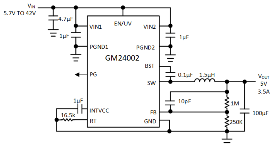
图 8. 2MHz, V_{IN}=12V , V_{OUT}=5V , I_{LOAD}=3.5A
