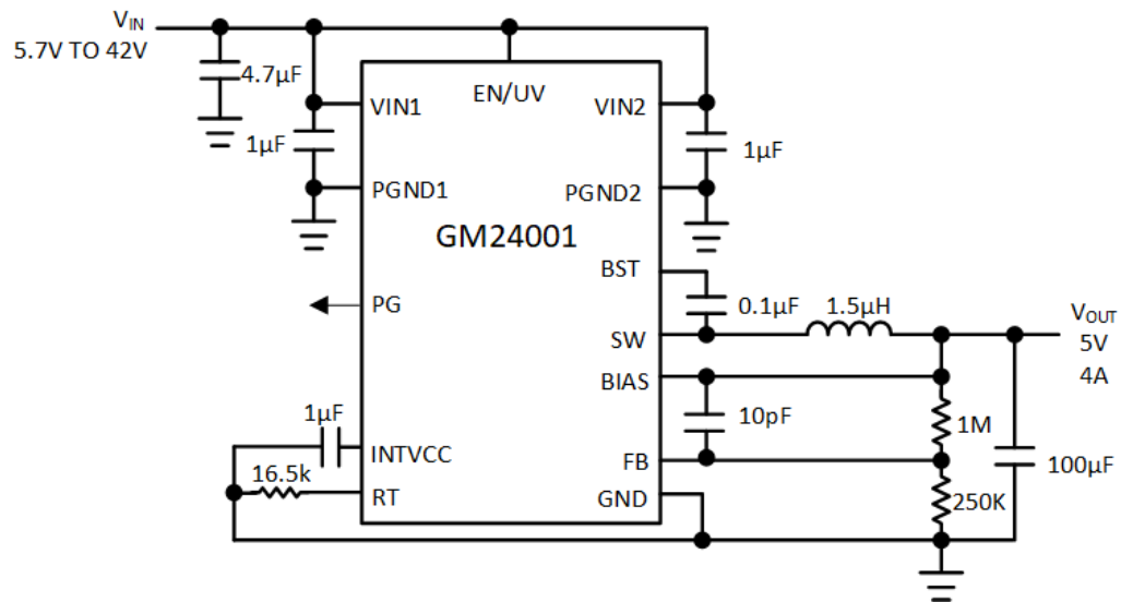
图 7. 2MHz, V_{IN}=12V , V_{OUT}=5V , I_{LOAD}=4A
