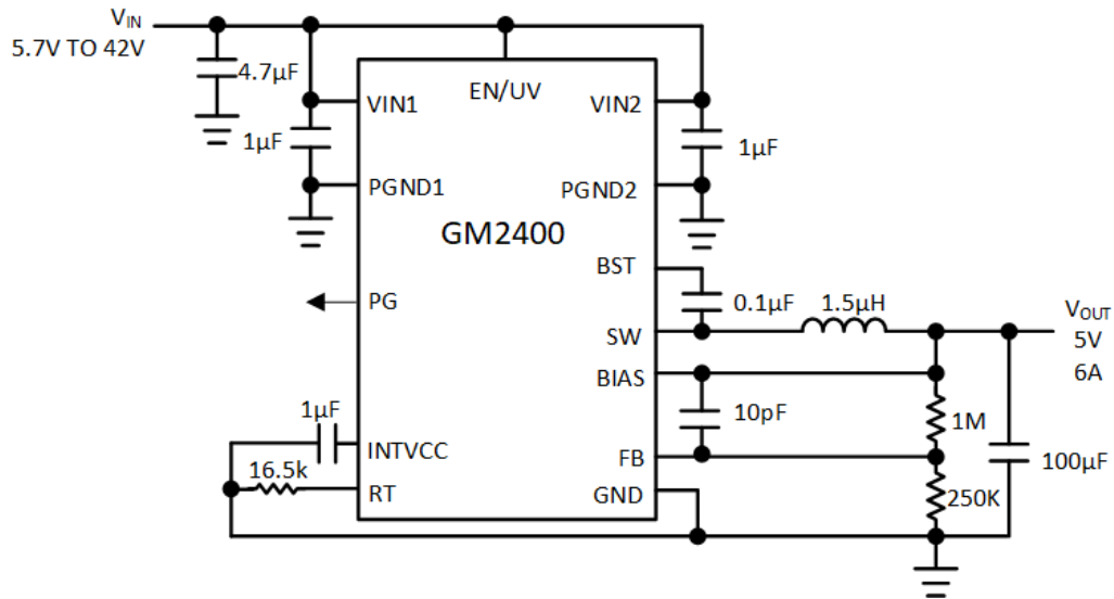
图 6. 2MHz, V_{IN}=12V , V_{OUT}=5V , I_{LOAD}=6A
