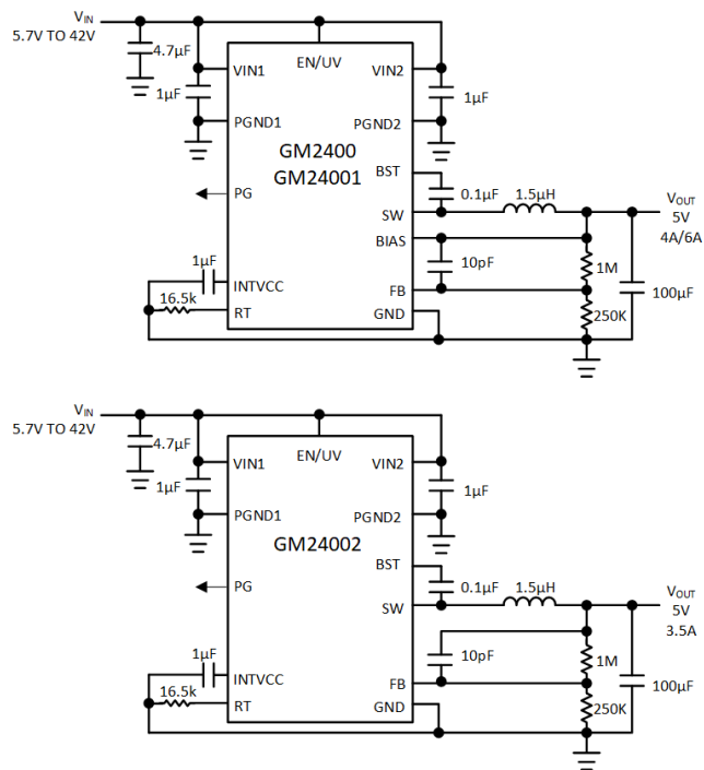
图 1. 2MHz 典型应用
