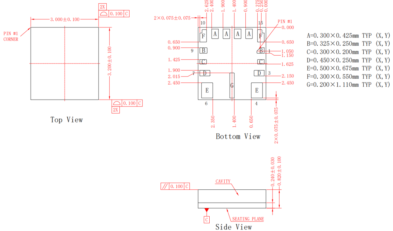
图 10.15 引脚 QFN
