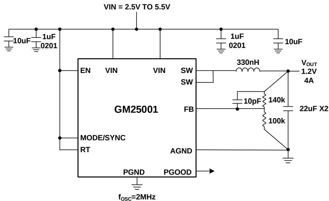
图 32. 2MHz, V_{IN}=3.3V , V_{OUT}=1.2V , I_{LOAD}=4A
