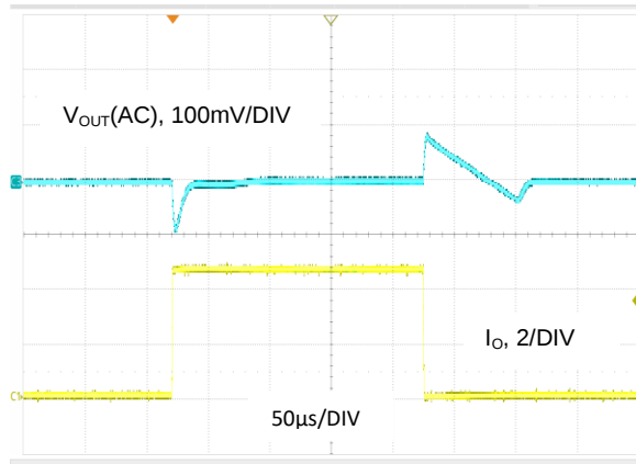
图 24. V_{OUT} = 1.2V , I_O = 0.1A 至 4.5A , PSM 模式
