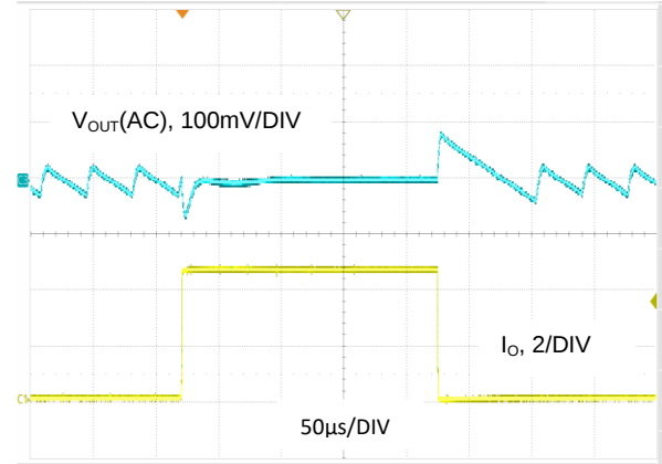
图 25. V_{OUT} = 1.2V , I_O = 0.1A 至 4.5A , 低功耗模式
