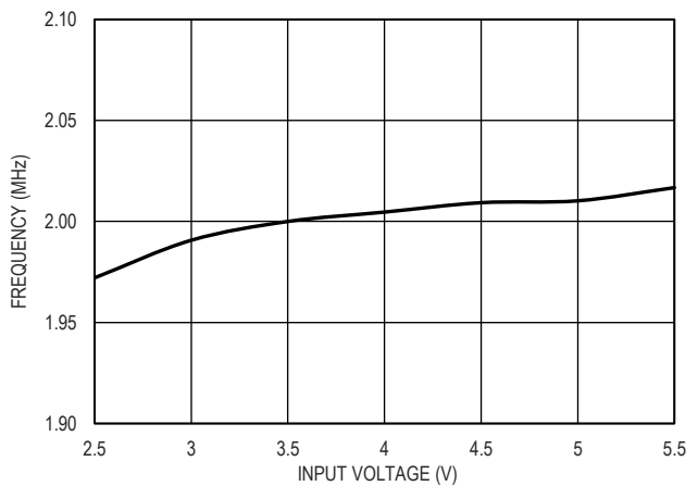
图 11. 频率和输入电压的关系, RT 接高
