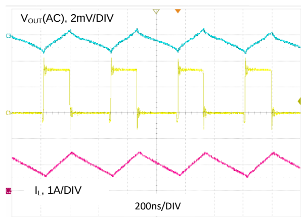
图 20. V_{OUT} = 1.2V , I_O = 1A , FPWM
