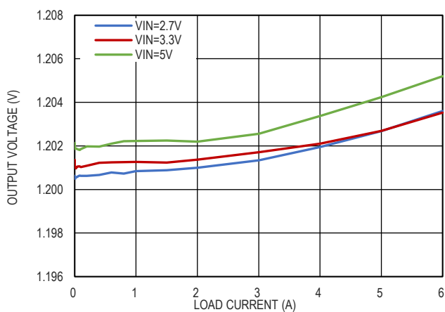
图 14. 输出电压负载调整率, V_{OUT} = 1.2V
