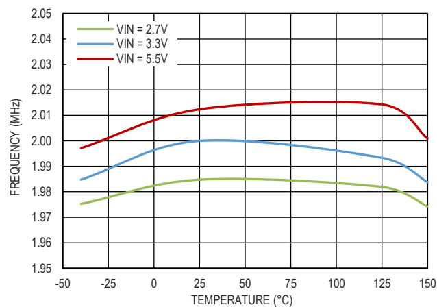
图 13. 频率和温度的关系, RT 接高
