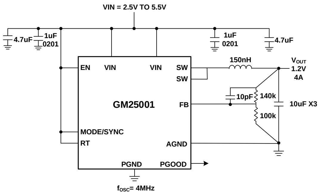
图 33. 4MHz, V_{IN}=3.3V , V_{OUT}=1.2V , I_{LOAD}=4A
