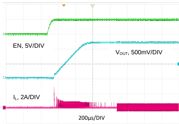
图 18. 启动波形, V_{OUT} = 1.2V , I_O = 10mA
