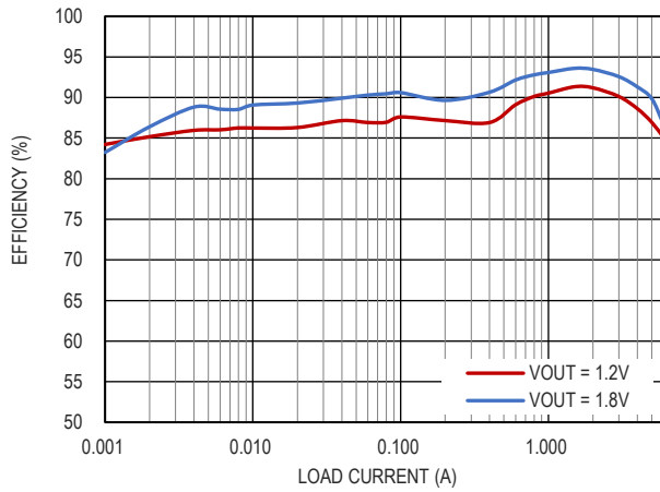
图 6. 效率曲线, V_{IN} = 3.3V , F_{SW} = 2MHz , 低功耗模式
