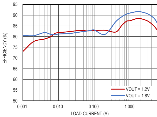
图 8. 效率曲线, V_{IN} = 3.3V , F_{SW} = 4MHz , 低功耗模式
