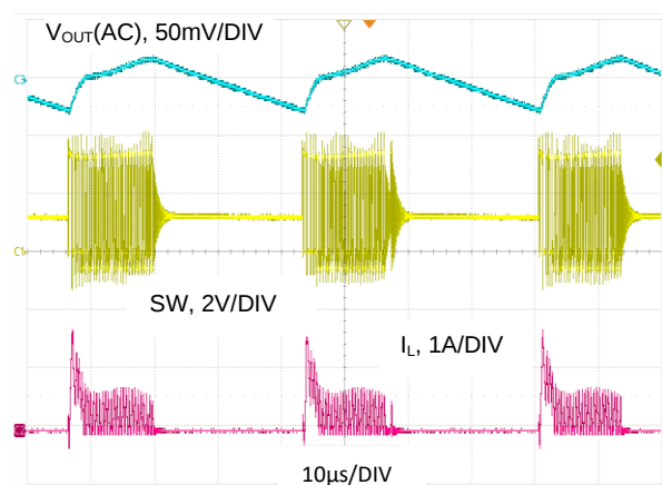
图 22. V_{OUT} = 1.2V , I_O = 10mA , 低功耗模式
