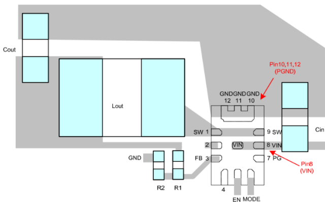
图 28. GM25002 PCB 推荐布局
