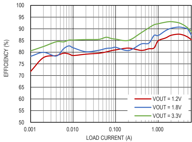
图 9. 效率曲线, V_{IN} = 5V , F_{SW} = 4MHz , 低功耗模式
