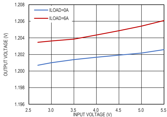
图 15. 输出电压线调整率, V_{OUT} = 1.2V
