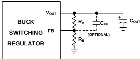
图 26. 反馈电阻网络
