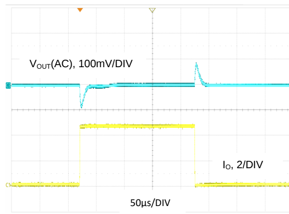
图 23. V_{OUT} = 1.2V , I_O = 0.1A 至 4.5A , FPWM 模式
