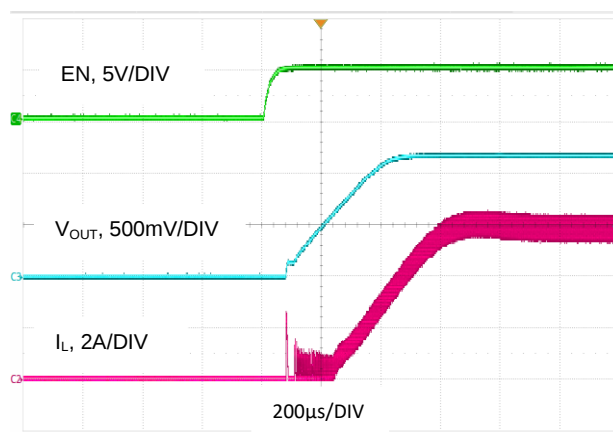
图 19. 启动波形, V_{OUT} = 1.2V , I_O = 6A
