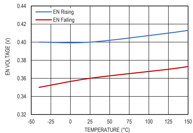
图 16. EN 阈值和温度的关系
