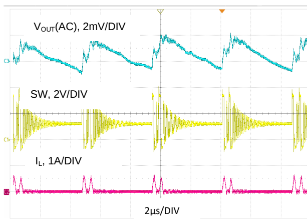
图 21. V_{OUT} = 1.2V , I_O = 100mA , PSM 模式
