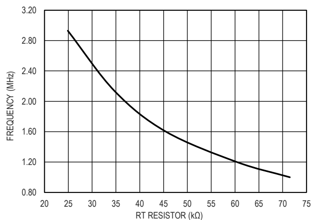
图 12. 频率和 RT 电阻的关系
