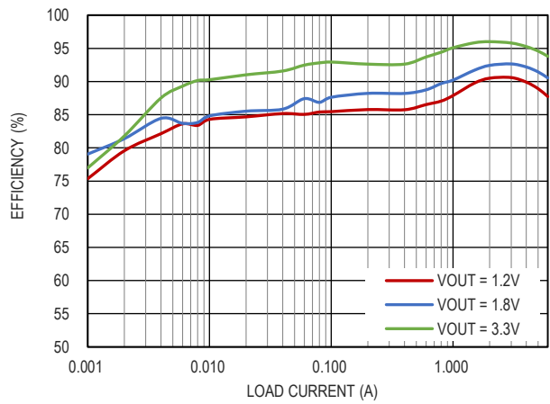
图 7. 效率曲线, V_{IN} = 5V , F_{SW} = 2MHz , 低功耗模式
