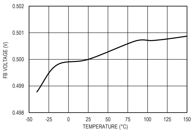
图 10. FB 引脚电压和温度的关系
