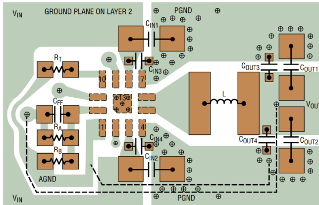
图 27. GM2500 和 GM25001 PCB 推荐布局
