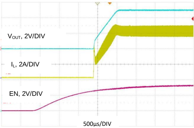
图 10. 启动波形, V_{OUT} = 1.2V , I_O = 2A
