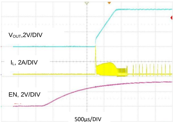
图 9. 启动波形, V_{OUT} = 1.2V , I_O = 10mA
