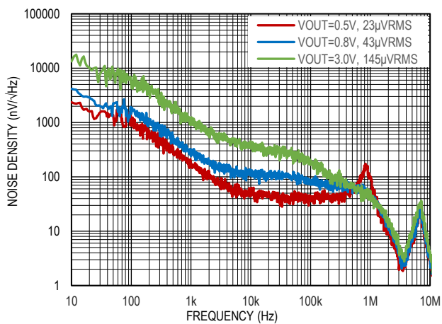
图 17. 输出噪声谱密度
