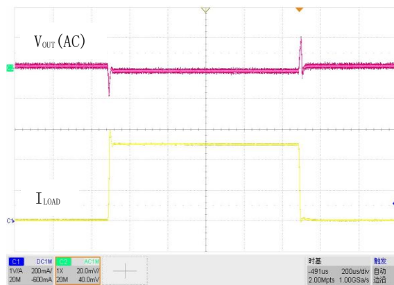
图 22. 负载瞬态响应, V_{IN}=1.2V , V_{OUT}=0.8V , I_{OUT}=1mA to 500mA
