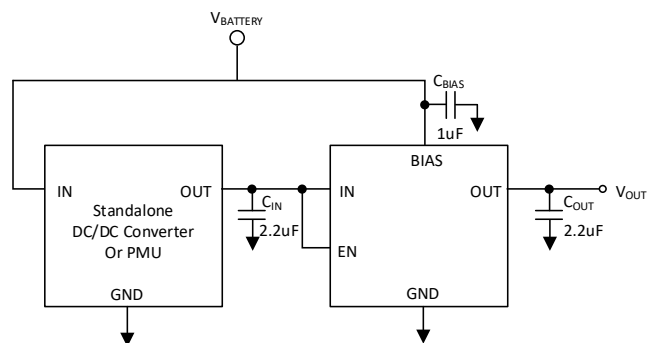
典型应用
