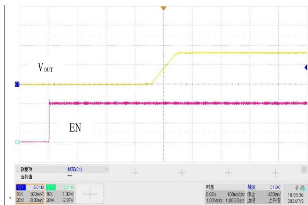
图 21. 软启动, V_{IN}=1.2V , V_{OUT}=0.8V , I_{OUT}=2A
