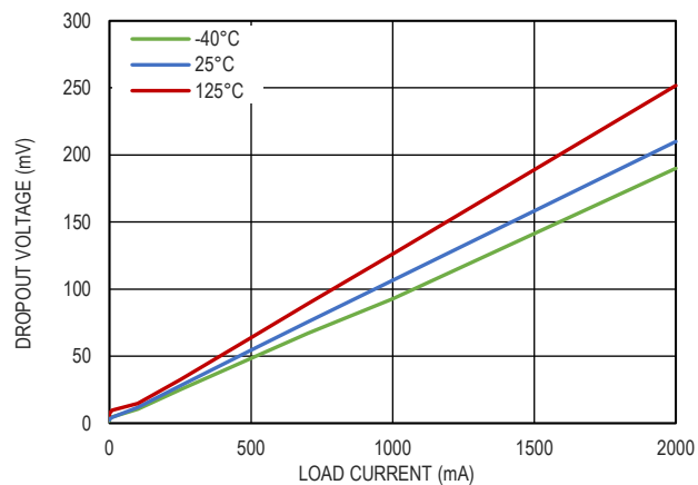
图 5. 压差电压和负载电流的关系, V_{OUT}=0.8V
