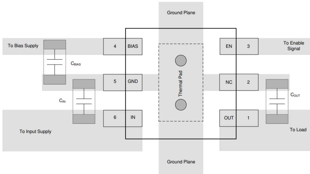
图 23. 版图示例
