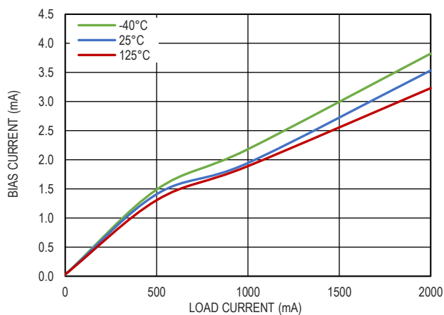
图 8. BIAS 静态电流和负载电流的关系, V_{OUT}=0.8V
