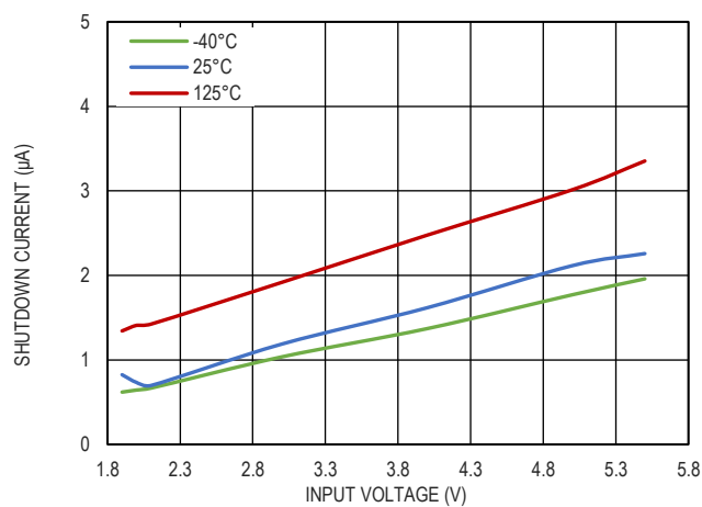
图 12. BIAS 关机电流和输入电压的关系
