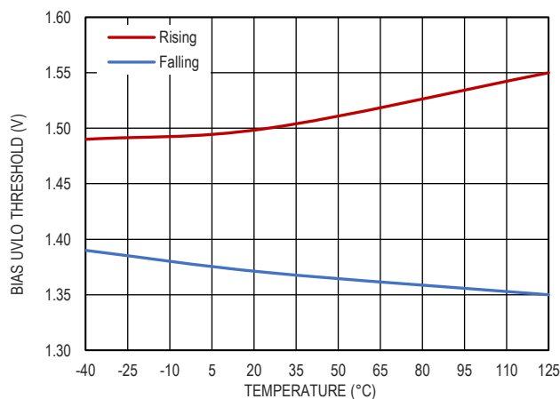
图 16. BIAS UVLO 阈值和温度的关系
