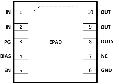
DFN 10-LEAD (3mmx3mm) 裸露焊盘必须焊接到 PCB 上
