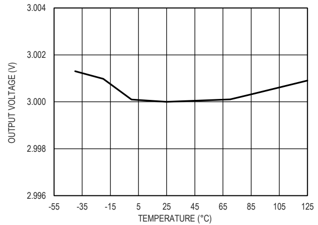
图 7. 2.048V 输出电压和温度的关系
