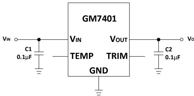
图 26. 有电容的应用电路
