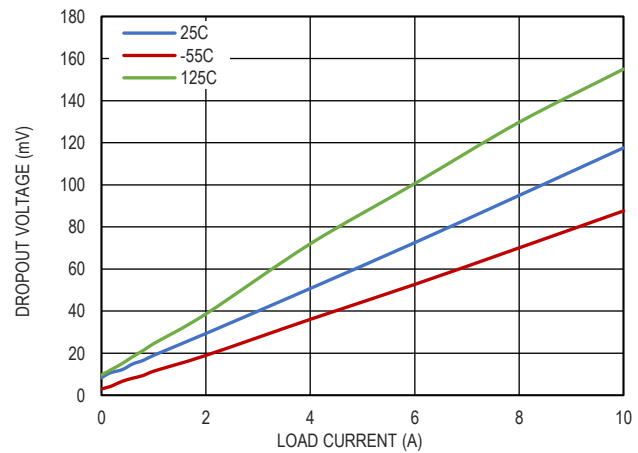
图 25. 最小输入电压和输出电压的关系, V_{OUT}=4.096V
