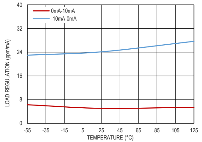
图 13. 负载调整率和温度的关系, V_{OUT}=4.096V
