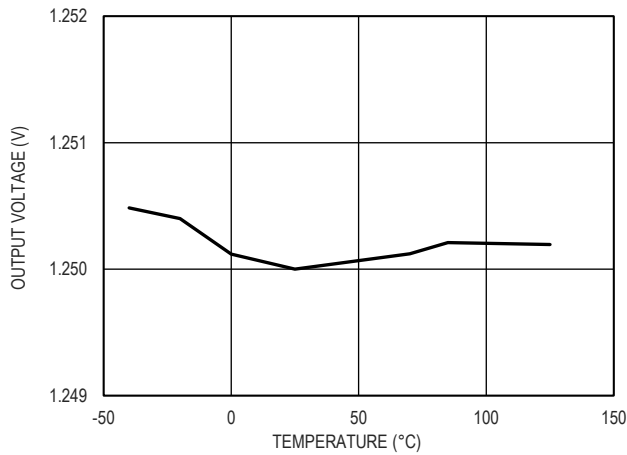
图 6. 1.25V 输出电压和温度的关系
