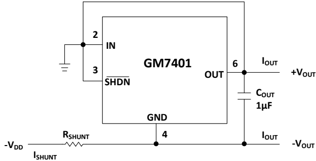
图 29. 负压并联方式
