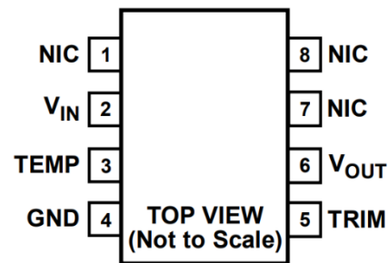
图 2. 8 引脚 SOIC
