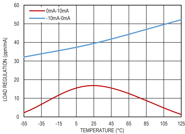
图 10. 负载调整率和温度的关系, V_{OUT}=1.25V
