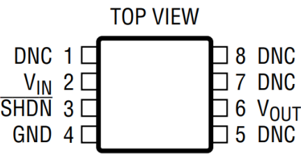
图 3. MSOP-8 引脚配置(顶视图, GM7400)
