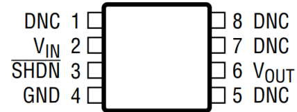
图 1. 8 引脚 MSOP
