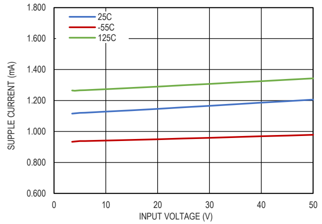
图 19. 输入电流和输入电压的关系, V_{OUT}=2.048V
