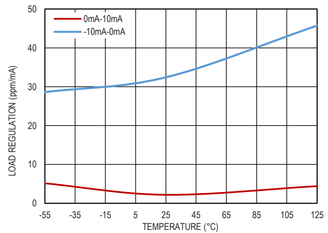
图 11. 负载调整率和温度的关系, V_{OUT}=2.048V
