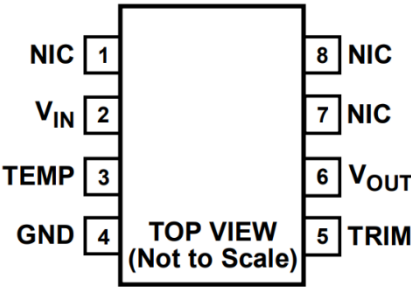
图 5. SO-8 引脚配置(顶视图)
