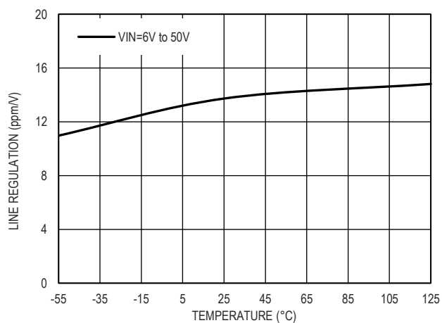
图 16. 输入调整率和温度的关系, V_{OUT}=3.3V
