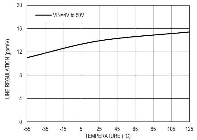
图 15. 输入调整率和温度的关系, V_{OUT}=2.048V
