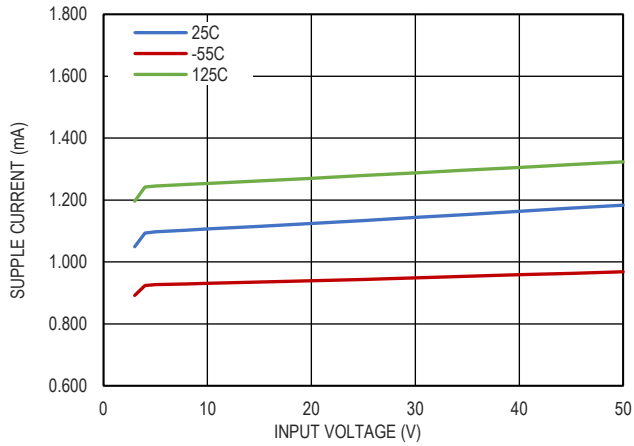
图 18. 输入电流和输入电压的关系, V_{OUT}=1.25V
