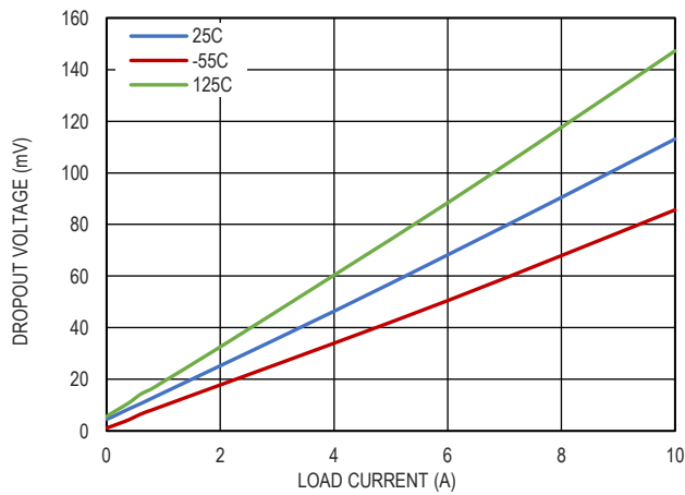
图 24. 最小输入电压和输出电压的关系, V_{OUT}=3.3V
