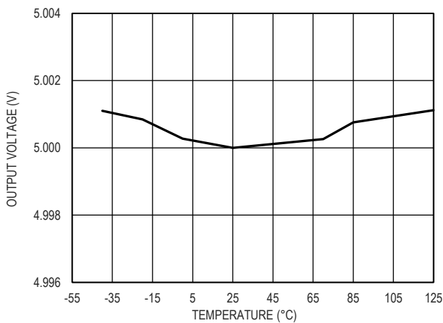
图 8. 3.3V 输出电压和温度的关系
