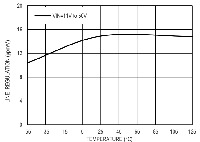
图 17. 输入调整率和温度的关系, V_{OUT}=4.096V
