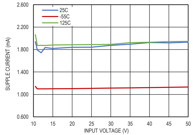
图 21. 输入电流和输入电压的关系, V_{OUT}=4.096V
