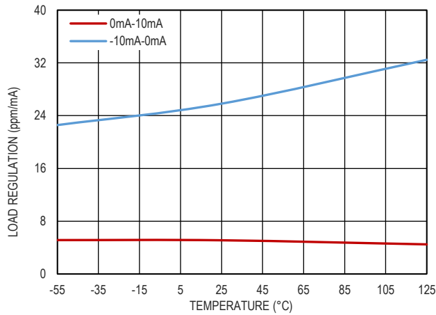
图 12. 负载调整率和温度的关系, V_{OUT}=3.3V
