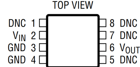
图 4. MSOP-8 引脚配置(顶视图, GM7400-1)
