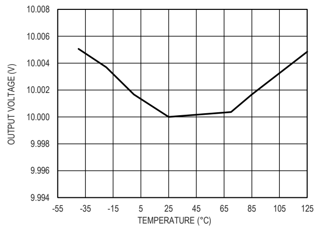
图 9. 4.096V 输出电压和温度的关系
