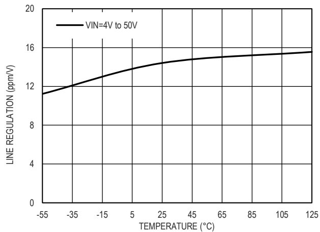
图 14. 输入调整率和温度的关系, V_{OUT}=1.25V
