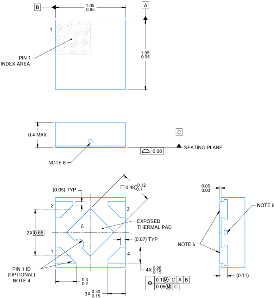
图 26.4 脚 DFN-4
