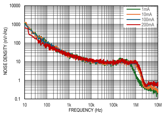
图 18. 输出噪声谱密度, V_{IN}=5V , V_{OUT}=3.6V
