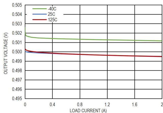
图 4. 负载调整率
