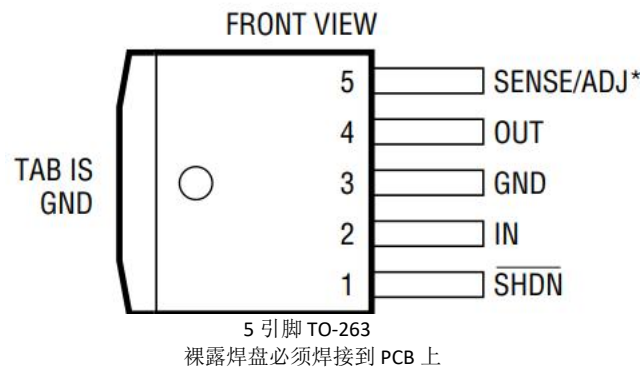
图 2 引脚配置
