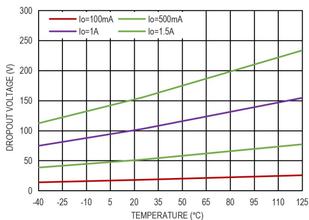
图 5. 压差电压和温度的关系
