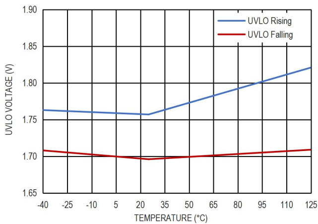
图 14. UVLO 阈值
