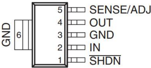
5 引脚 SOT-223 裸露焊盘必须焊接到 PCB 上 图 3 引脚配置
