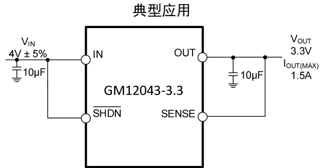
图 1 典型应用
