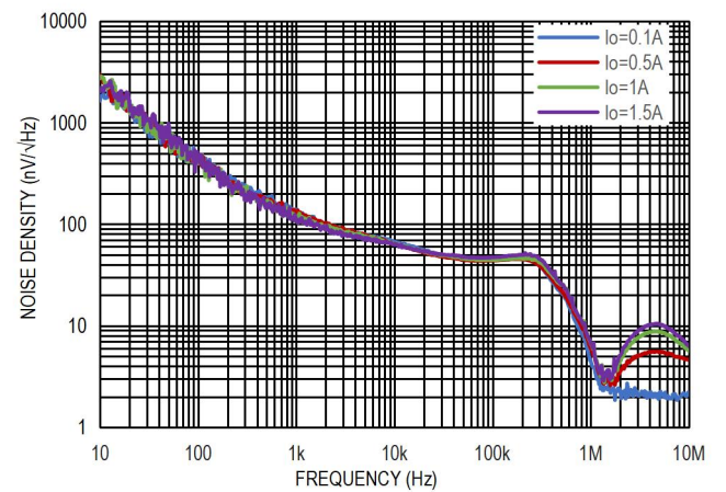
图 15. 输出噪声谱密度, V_{IN}=5V , V_{OUT}=3.3V
