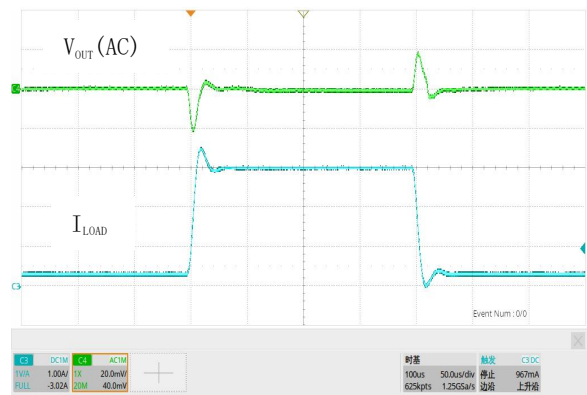
图 19. 负载瞬态响应, V_{IN}=2.8V , V_{OUT}=1.8V , I_{OUT}=0.1A to 1.5A
