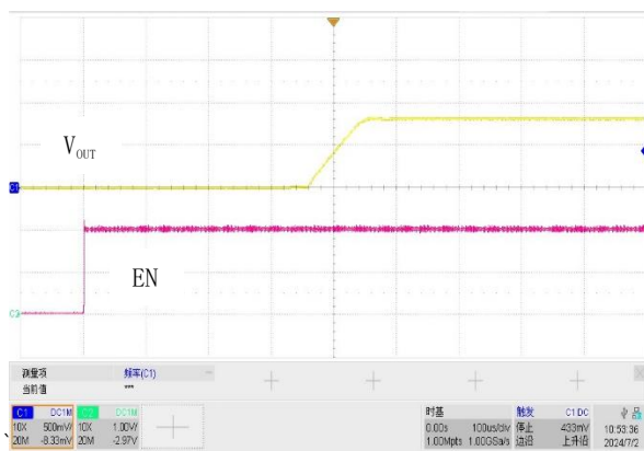
图 20. 软启动, V_{IN}=1.2V , V_{OUT}=0.8V , I_{OUT}=500mA
