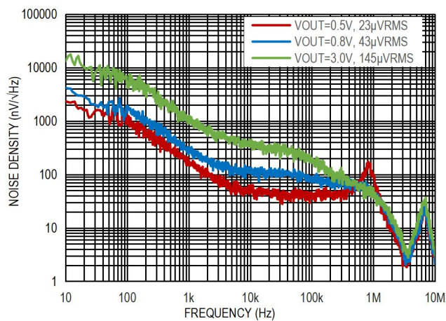
图 16. 输出噪声谱密度
