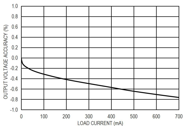
图 12. 输出电压精度和负载电流的关系
