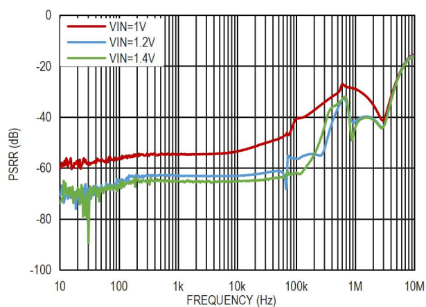
图 18. 电源电压纹波抑制比与压差的关系, V_{OUT}=0.8V
