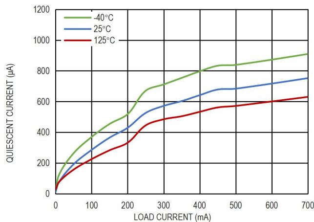
图 9. V_{IN} 静态电流和负载电流的关系, V_{OUT}=0.8V
