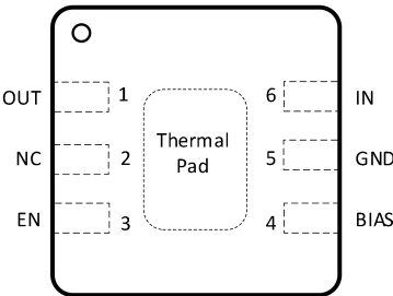
Not to scale DFN 6-LEAD (2mm×2mm) 裸露焊盘必须焊接到 PCB 上 图 3 引脚配置
