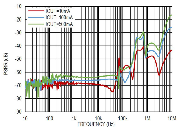
图 19. 电源电压纹波抑制比与负载的关系, V_{OUT}=0.8V
