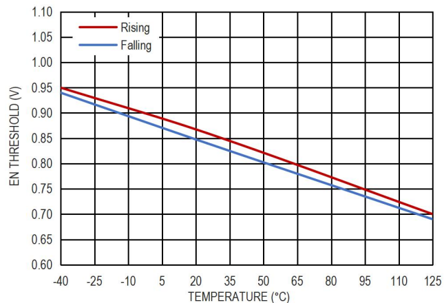
图 13. EN 阈值和温度的关系
