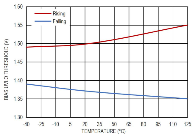
图 15. BIAS UVLO 阈值和温度的关系
