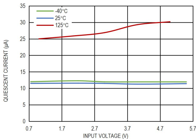
图 8. V_{IN} 静态电流和输入电压的关系, I_{OUT} = 0mA
