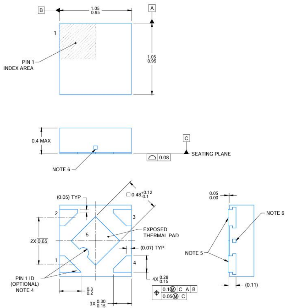
图 26.4 脚 DFN-4
