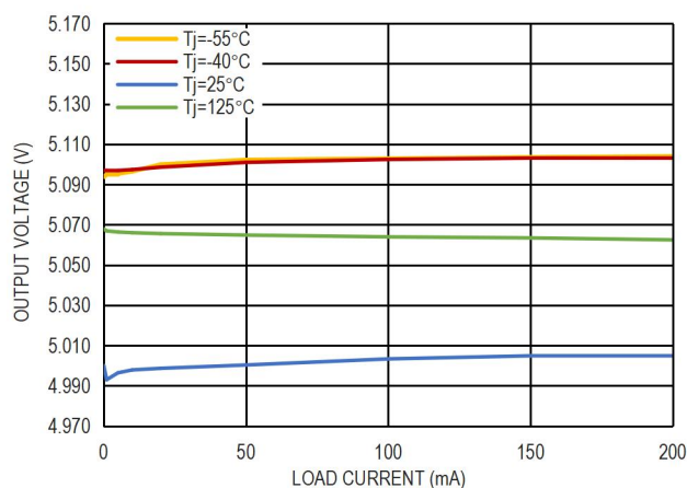
图 13. 5.0V 输出电压和负载电流的关系
