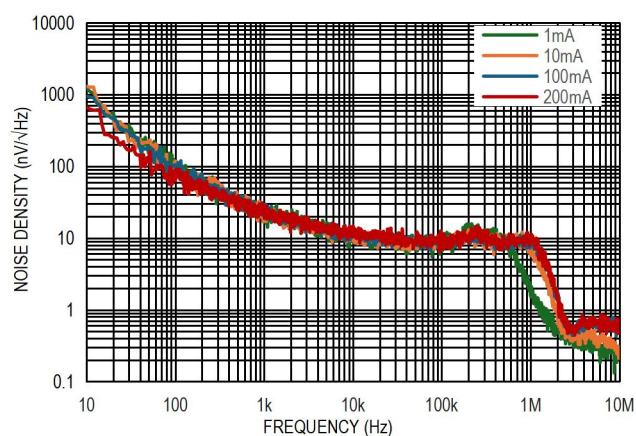
图 18. 输出噪声谱密度, V_{IN}=5V , V_{OUT}=3.6V
