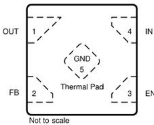
图 4.5 引脚 DFN-5 引脚配置（可调输出）
