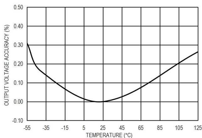
图 15. 固定输出电压精度
