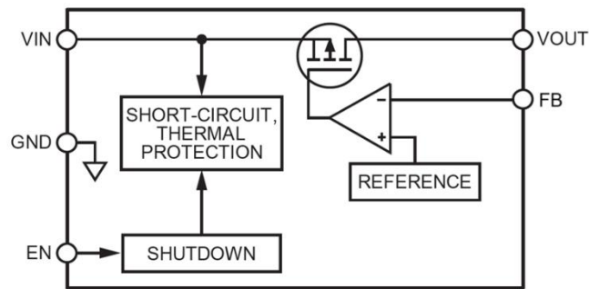
图 23. 内部框图
