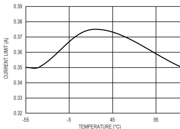
图 16. 输出限流值和温度的关系
