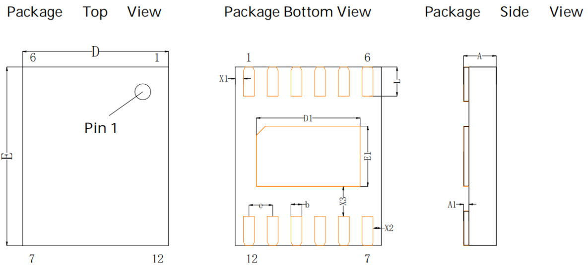
图 30. DFN12 封装 (4mmx4.9mm, CP-12-2) 和 MSOP-12 管脚兼容
