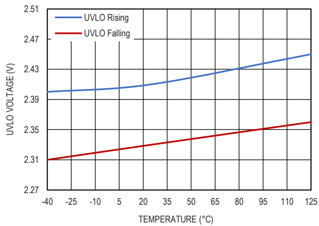
图 17. UVLO 阈值
