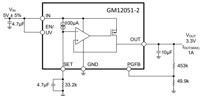
图 2 典型应用
