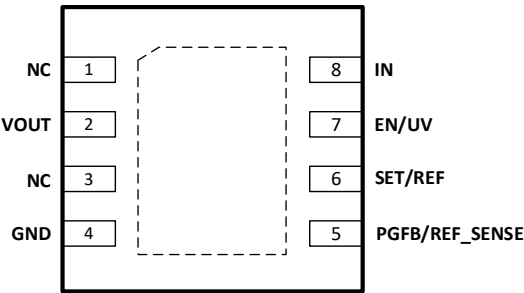
图 7. GM12051ACPZ-2 引脚配置(顶视图)
