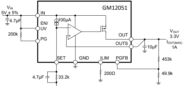
图 26 典型应用
