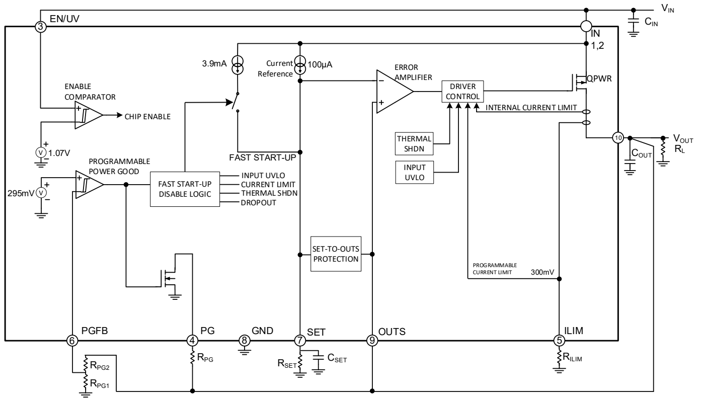
图 3 GM12051 功能框图
