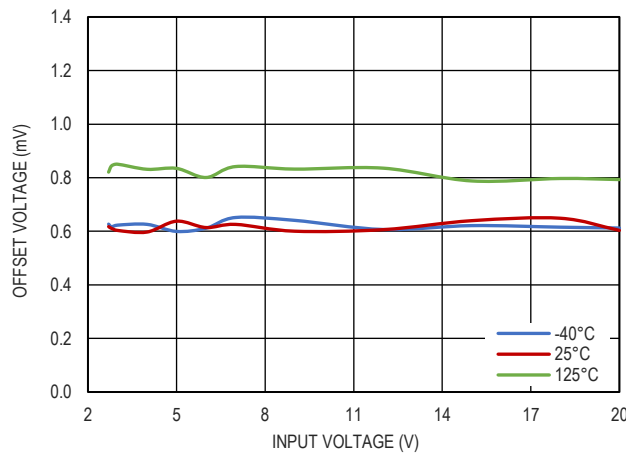
图 10. |V_{OUT}-V_{SET}| 和输入电压的关系, V_{OUT}=1.8V
