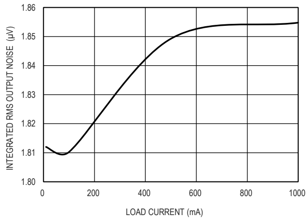
图 22. 积分 RMS 输出噪声, V_{IN}=5V , V_{OUT}=3.3V
