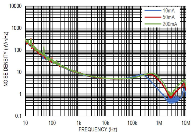
图 17. 输出噪声谱密度, V_{IN}=4.3V , V_{OUT}=3.3V
