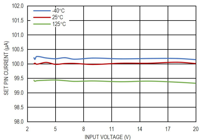
图 4. SET pin 电流和输入电压的关系
