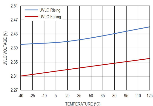
图 13. UVLO 阈值
