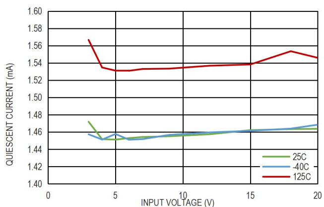
图 10. 静态电流和输入电压的关系, I_{OUT}=10mA
