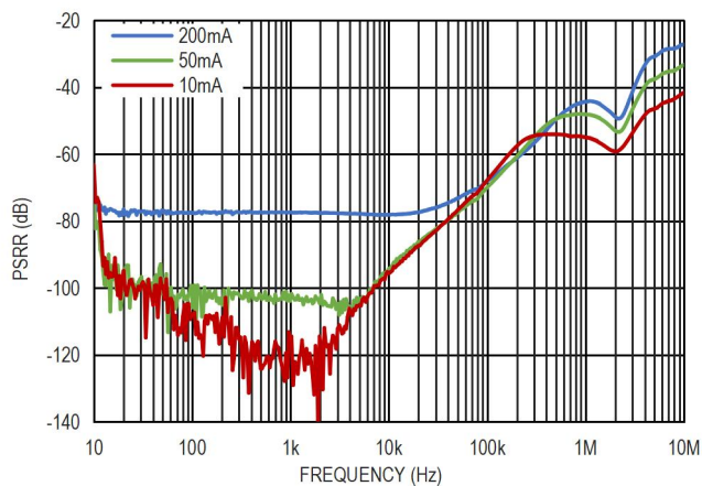
图 18. 电源电压纹波抑制比, V_{IN}=4.1V , V_{OUT}=3.6V
