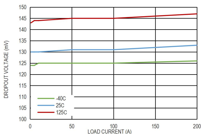
图 12. 压差电压和负载电流的关系, V_{OUT}=5.0V
