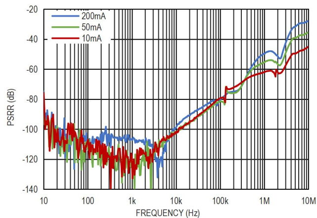
图 19. 电源电压纹波抑制比, V_{IN}=4.6V , V_{OUT}=3.6V
