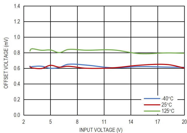
图 6. |V_{OUT}-V_{SET}| 和输入电压的关系, V_{OUT}=3.0V
