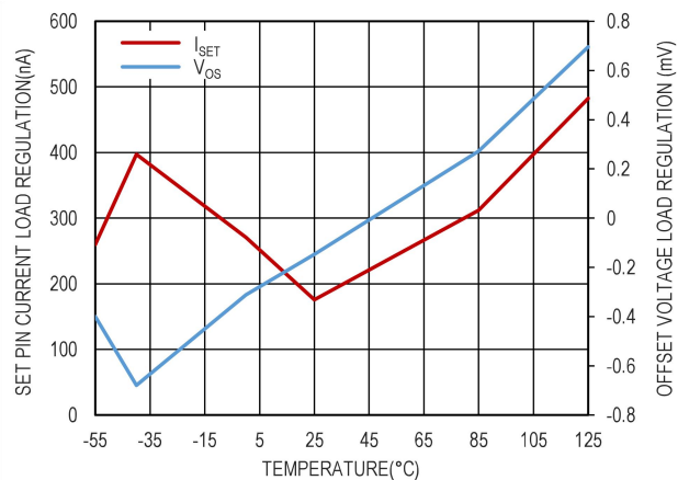
图 8. SET pin 电流、 |V_{OUT}-V_{SET}| 和温度的关系
