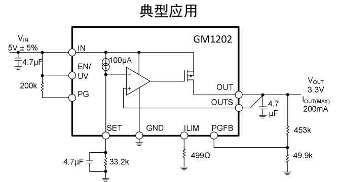
图 1 典型应用
