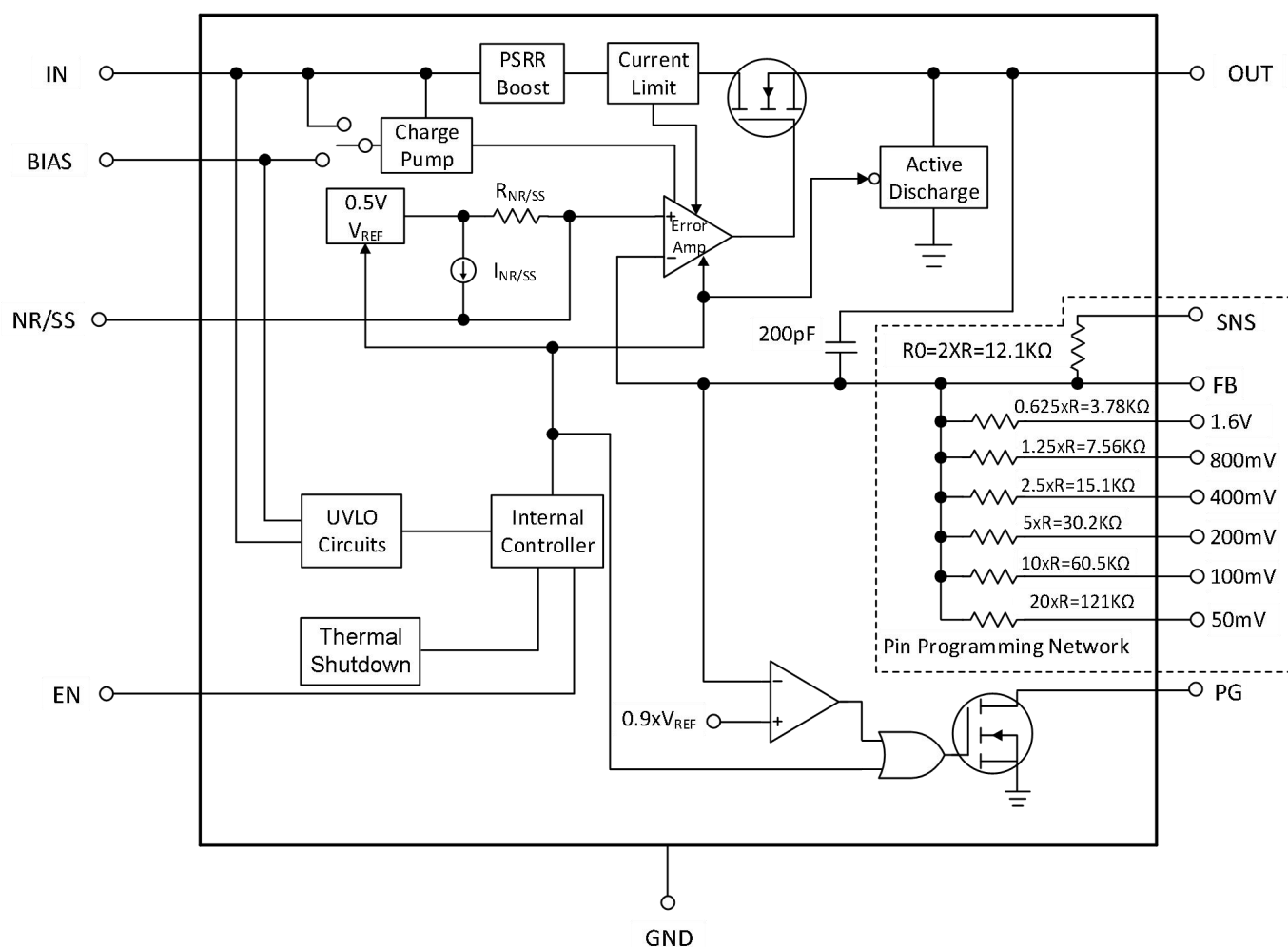
图 3. GM1503-1 方框图
