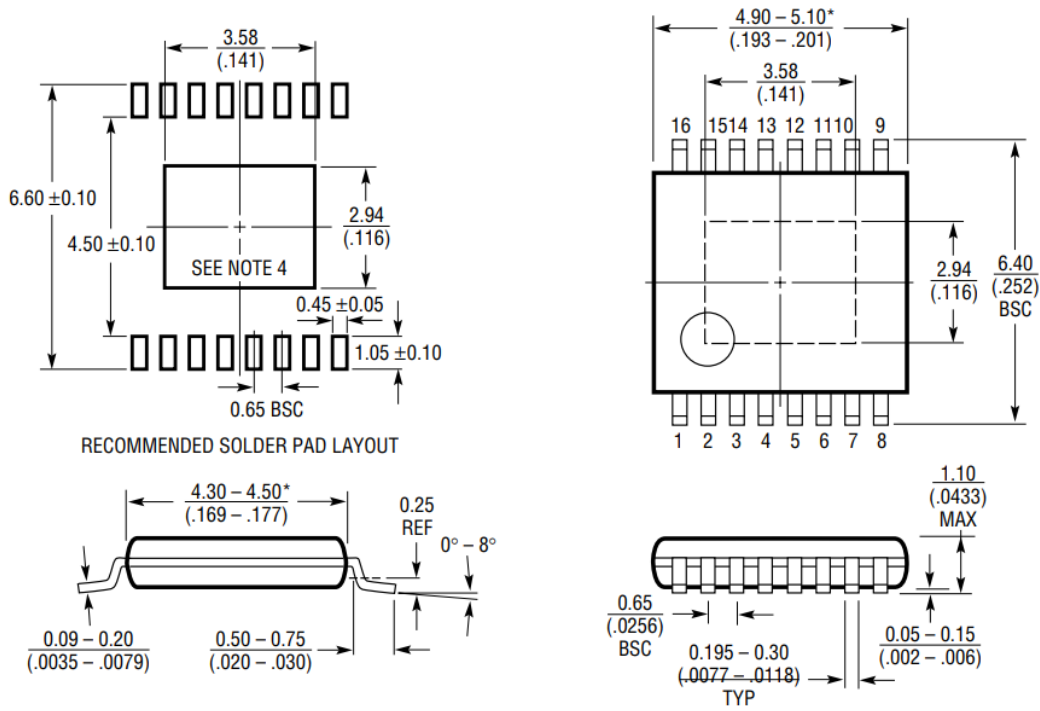
图 22.16 引脚 TSSOP
