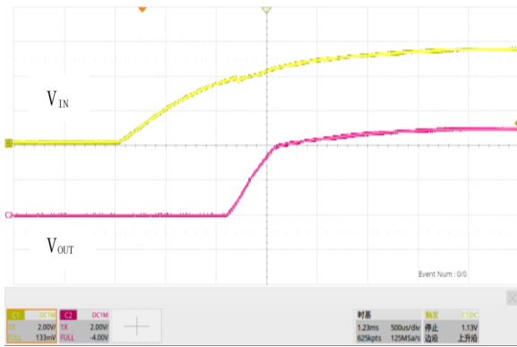
图 18. 软启动, V_{IN}=5.5V , V_{OUT}=5.0V , I_{OUT}=3A
