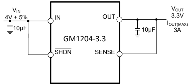
图 1 典型应用
