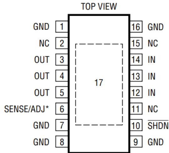
16 引脚 TSSOP
