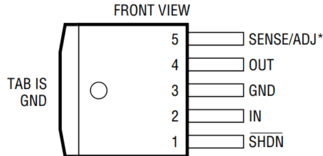
5 引脚 TO-263 裸露焊盘必须焊接到 PCB 上
