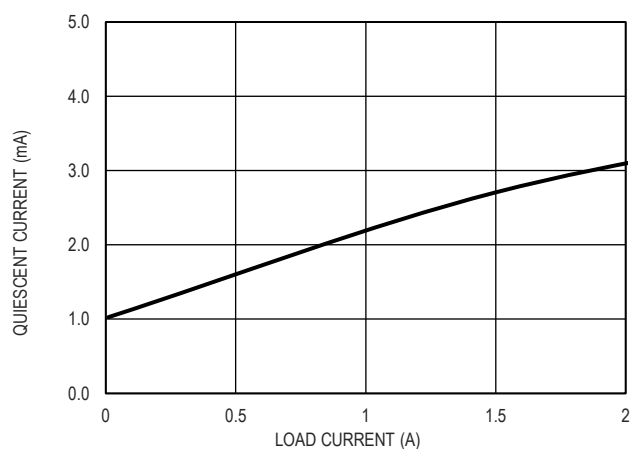
图 5. 静态电流和负载电流的关系
