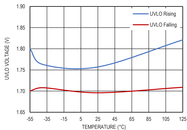
图 13. UVLO 阈值
