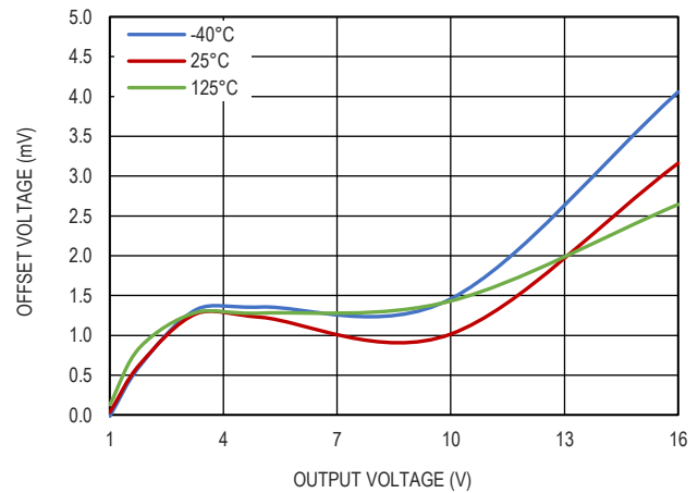
图 8. |V_{OUT}-V_{SET}| 和输出电压的关系
