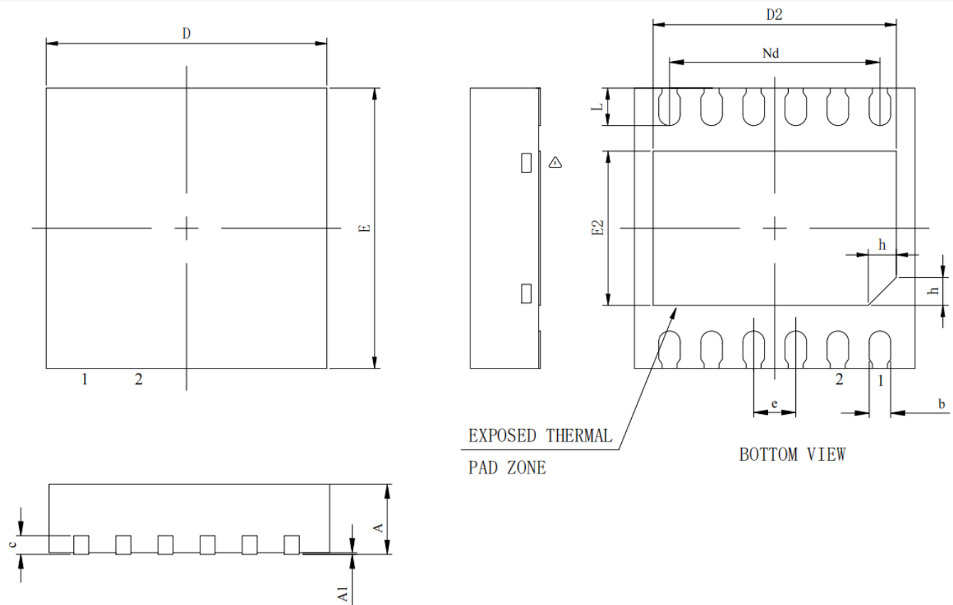
图 27. DFN12 封装 (3mmx3mm, CP-12-1)
