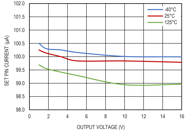
图 6. SET pin 电流和输出电压的关系
