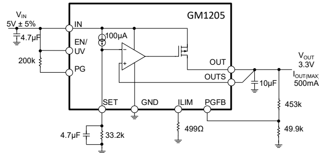
图 23 典型应用
