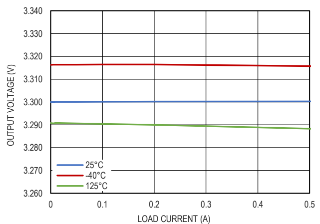
图 10. V_{OUT}=3.3V 时的负载调整率
