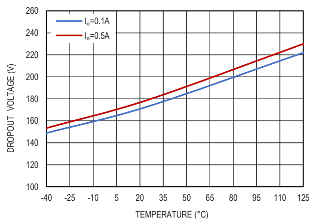
图 13. 压差电压和负载电流的关系, V_{OUT}=3.0V
