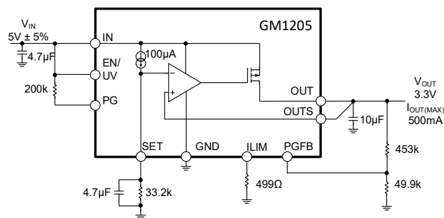
图 1. 典型应用
