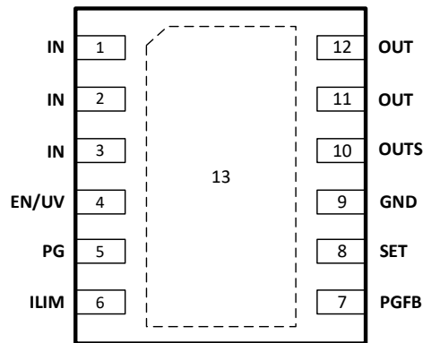
图 4.兼容 MSOP-12 的 4mmx4.9mm DFN12 引脚配置(顶视图)
