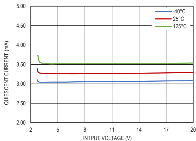
图 11. 静态电流和输入电压的关系, I_{OUT}=10mA
