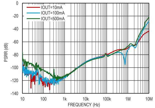
图 20. 电源电压纹波抑制比, V_{IN}=5V , V_{OUT}=3.3V
