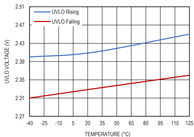
图 14. UVLO 阈值
