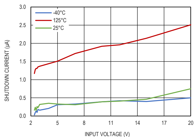
图 12. 停机静态电流和输入电压的关系
