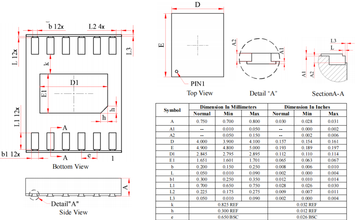
图 26. DFN12 封装 (4mmx4.9mm, CP-12-2) 和 MSOP-12 管脚兼容
