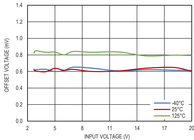
图 7. |V_{OUT}-V_{SET}| 和输入电压的关系, V_{OUT}=1.8V
