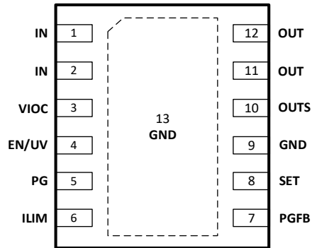
图 3. DFN12 (3mmx3mm 和 4mmx4.9mm 兼容 MSOP-12) 引脚配置(顶视图)
