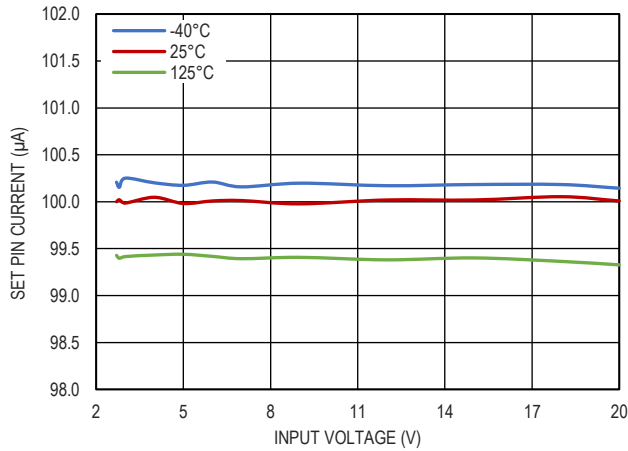
图 5. SET pin 电流和输入电压的关系
