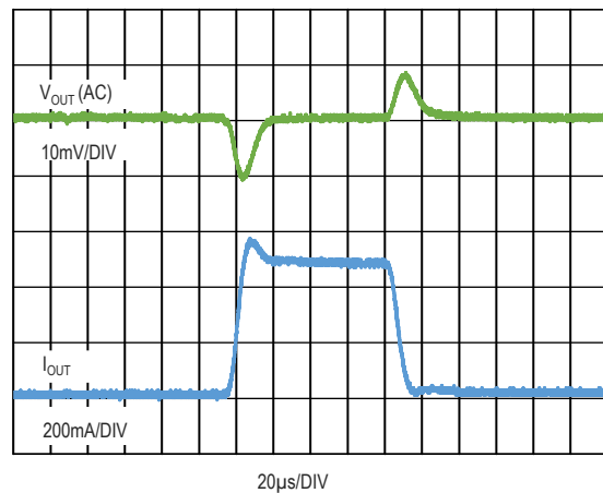
图 22. 负载瞬态响应, V_{IN}=4.3V , V_{OUT}=3.3V , I_{OUT}=1mA to 500mA
