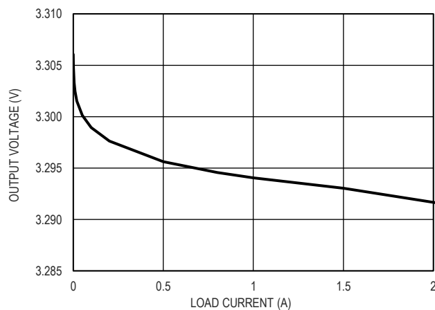
图 8. 3.3V 输出电压和负载电流的关系
