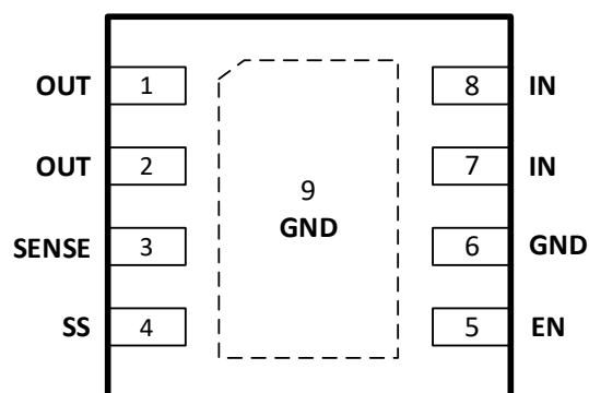
图 2 引脚配置
