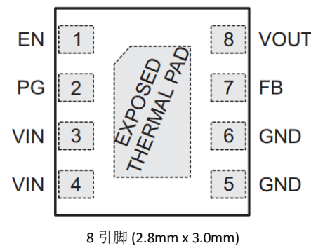
图 3 引脚配置 TOP VIEW
