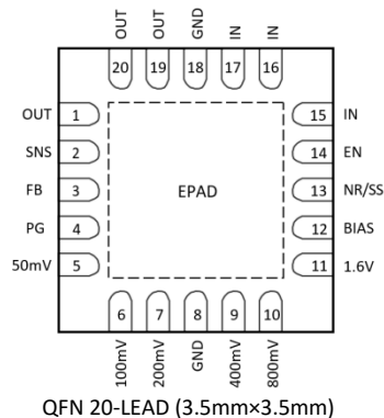
QFN 20-LEAD (3.5mm×3.5mm) 裸露焊盘必须焊接到 PCB 上
