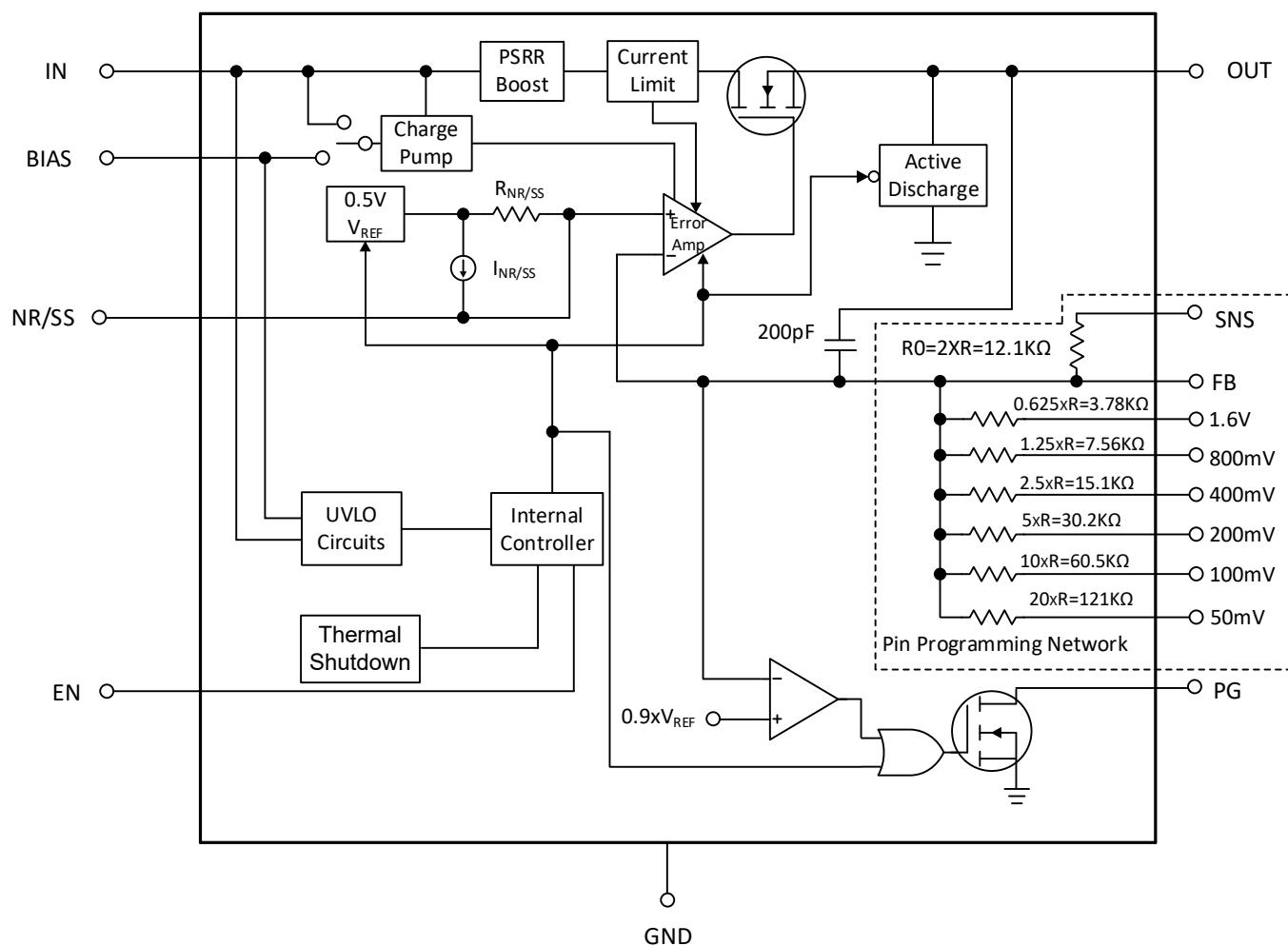
图 3. GM1203A-1 方框图
