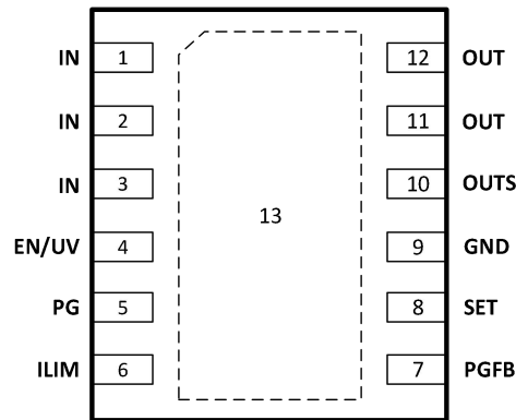
图 4.兼容 MSOP-12 的 4mmx4.9mm DFN12 GM1205ACPZ-3-R7 引脚配置(顶视图)
