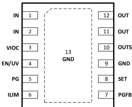
图 3. DFN12 (3mmx3mm GM1205ACPZ-2-R7 和 4mmx4.9mm GM1205ACPZ-1 兼容 MSOP-12) 引脚配置(顶视图)
