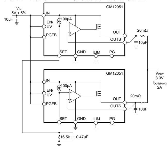
图 28. 并联设备
