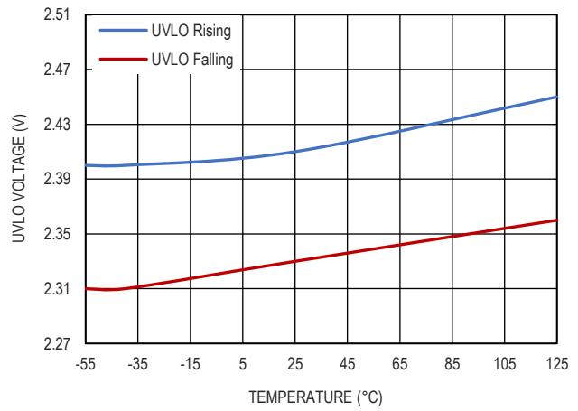
图 17. UVLO 阈值
