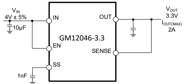
典型应用
