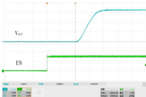
图 23. 软启动, V_{IN}=4.3V , V_{OUT}=3.3V , I_{OUT}=300mA
