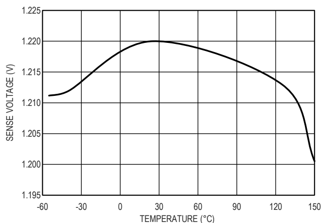
图 15. 1.22V SENSE 引脚电压精度
