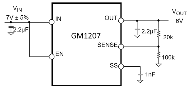
图 26. 典型可调输出电压应用原理图
