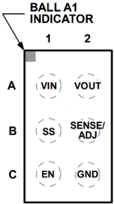
图 6.6 引脚 WLCSP 引脚配置
