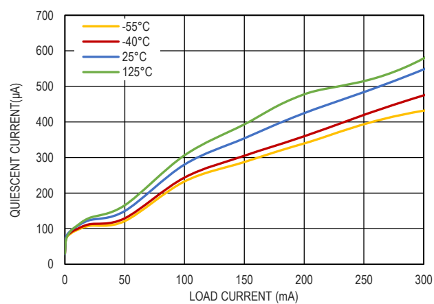
图 9. 静态电流和负载电流的关系, V_{IN}=4.3V
