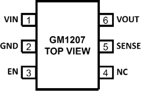
图 5.6 引脚 SOT-23 引脚配置
