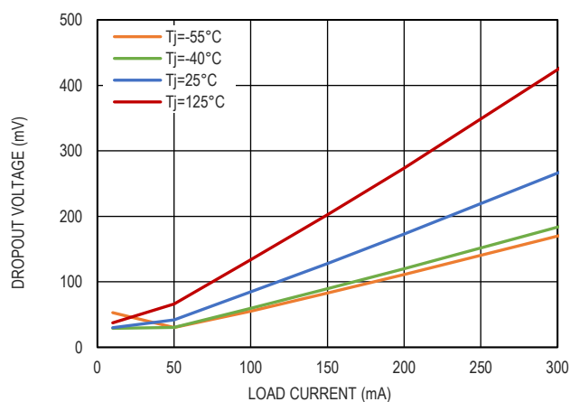
图 7. 3.3V 压差电压和负载电流的关系
