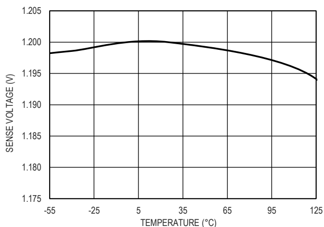
图 14. 1.2V SENSE 引脚电压精度
