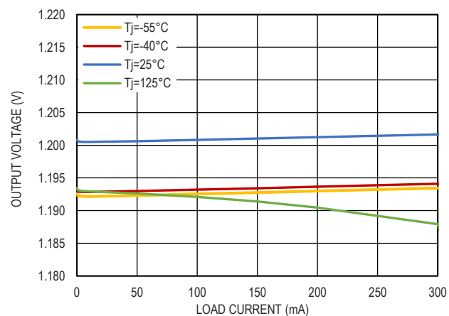
图 11. 1.2V 输出电压和负载电流的关系
