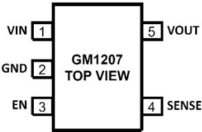
图 4.3 引脚 SOT-23 引脚配置
