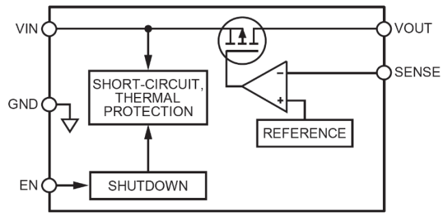
图 25. 内部框图
