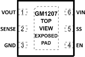
图 3.5 引脚 DFN-6 的引脚配置
