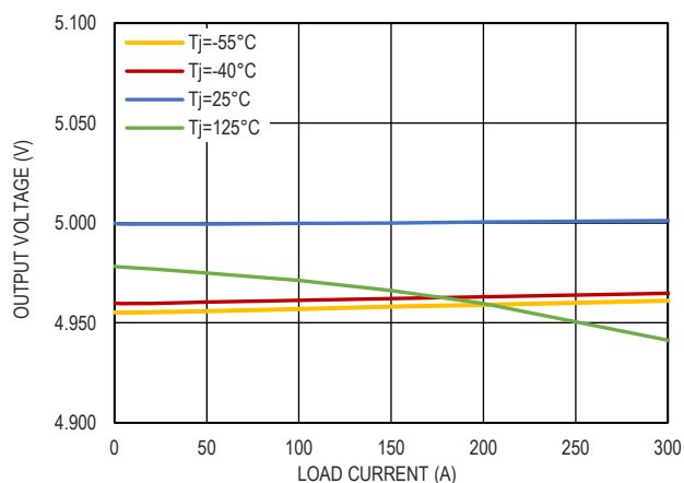
图 13. 5.0V 输出电压和负载电流的关系
