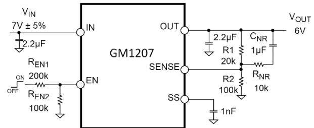
图 30. 噪声优化
