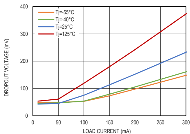
图 8. 5.0V 压差电压和负载电流的关系
