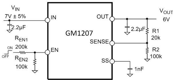
图 29. EN 引脚的典型分压器
