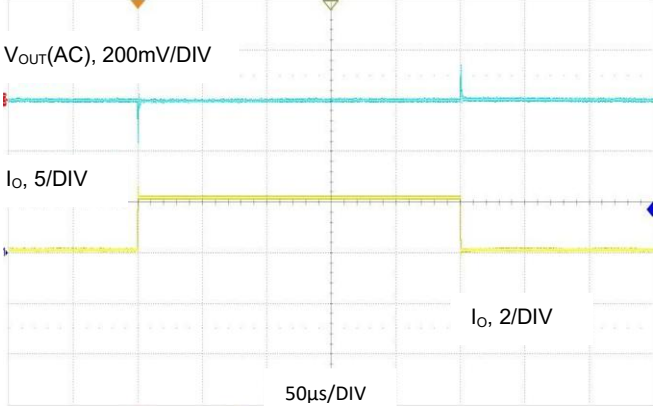
图 14. V_{OUT} = 5V , I_o = 0.2A 至 5.4A , FPWM 模式
