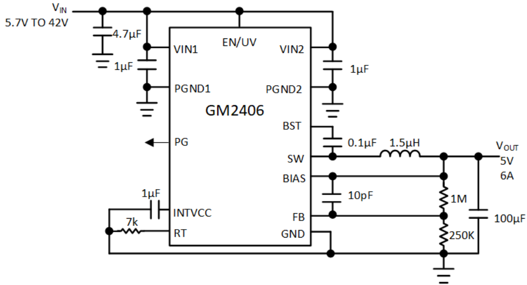
图 17. 2MHz, V_{IN}=12V , V_{OUT}=5V , I_{LOAD}=6A
