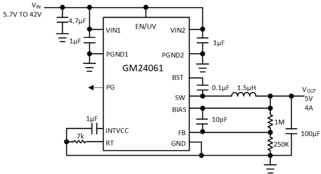
图 18. 2MHz, V_{IN}=12V , V_{OUT}=5V , I_{LOAD}=4A
