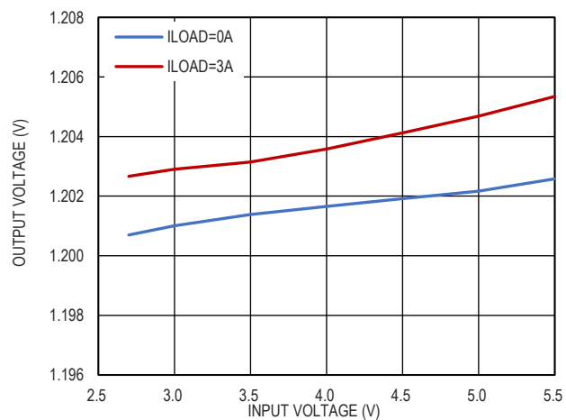
图 9. 输出电压线调整率, V_{OUT} = 1.2V
