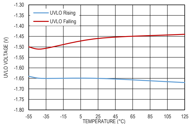
图 12. UVLO 阈值
