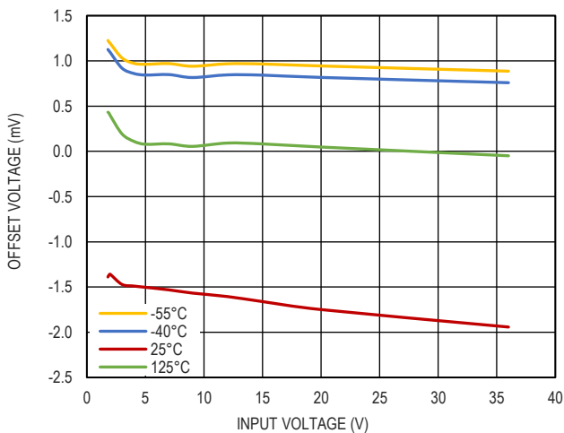
图 5. |V_{OUT}-V_{SET}| 和输入电压的关系, V_{OUT}=1.8V
