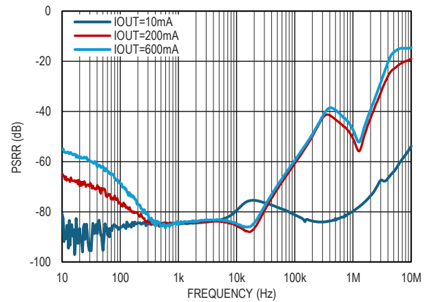
图 16. 电源电压纹波抑制比, V_{IN}=-4V , V_{OUT}=-3.3V
