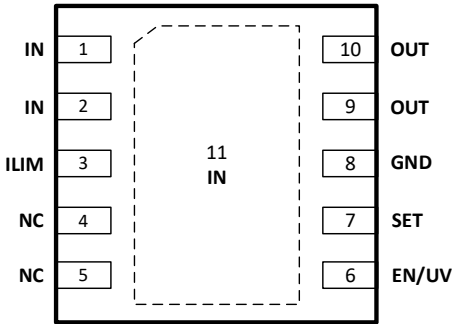
图 2. 引脚配置(顶视图)
