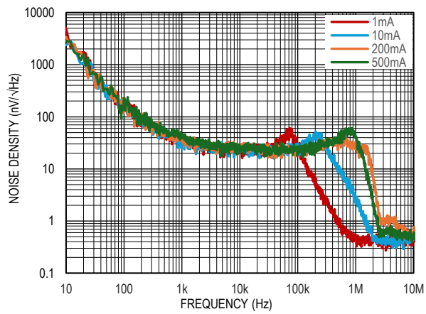
图 12. 噪声谱密度
