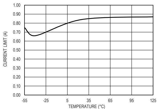
图 17. 限流值和结温的关系
