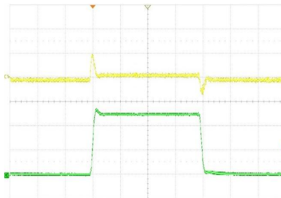
图 16. 负载瞬态响应, V_{IN} = -6V , V_{OUT} = -5V , I_O = -10 至 -500mA
