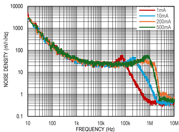
图 9. 噪声谱密度
