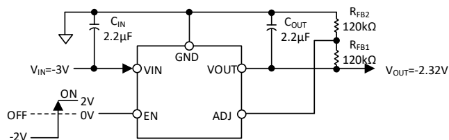
图 19. 设置可调输出电压
