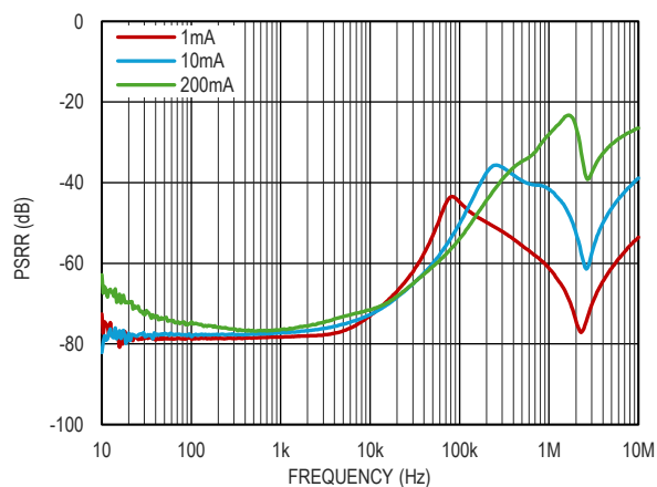
图 11. PSRR 和负载电流的关系
