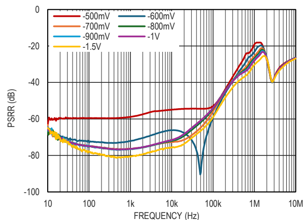
图 10. PSRR 和压差的关系, I_o = 500\text{mA}
