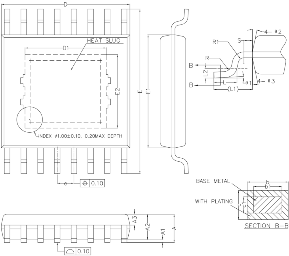
图 26.16 引脚 TSSOP
