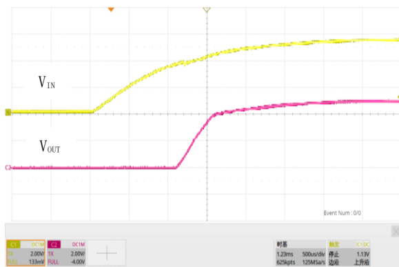
图 21. 软启动, V_{IN}=5.5V , V_{OUT}=5.0V , I_{OUT}=1.5A
