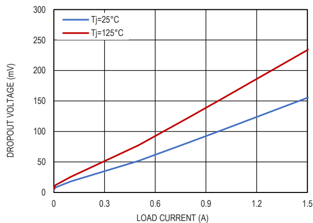
图 7. 压差电压和负载电流的关系
