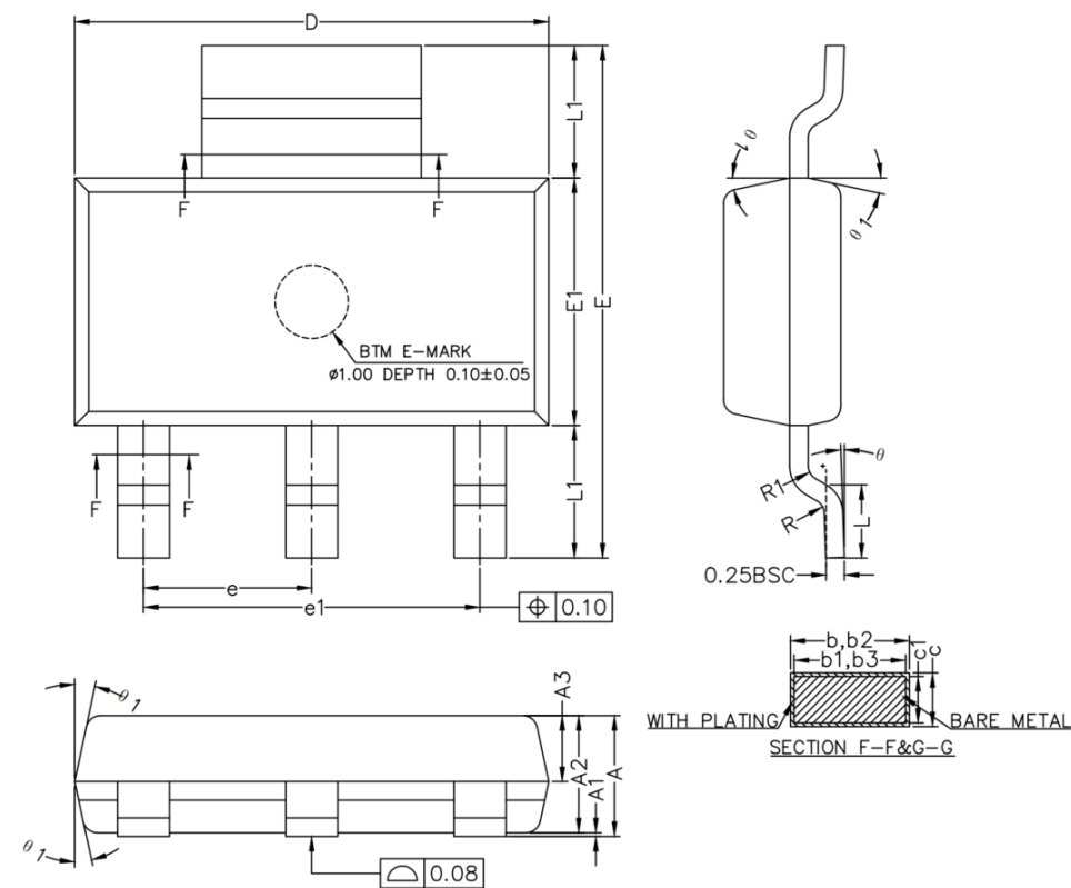
图 27.3 引脚 SOT-223
