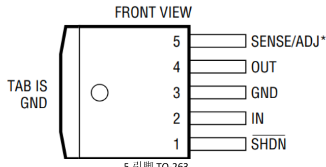
5 引脚 TO-263 裸露焊盘必须焊接到 PCB 上 图 2 引脚配置
