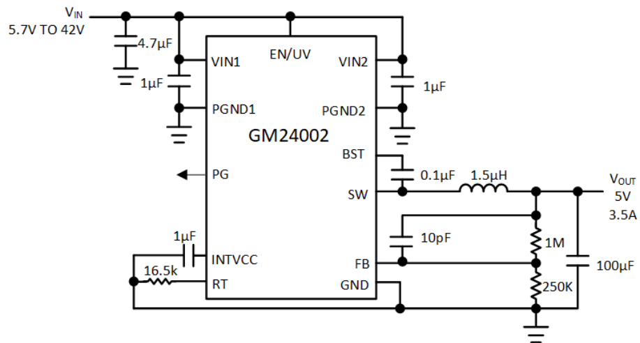
图 20. 2MHz, V_{IN}=12V , V_{OUT}=5V , I_{LOAD}=3.5A
