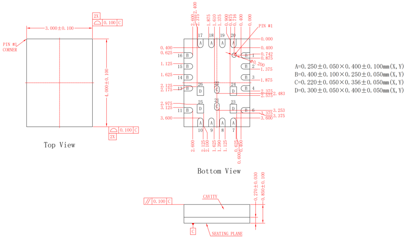
图 21.26 引脚 QFN
