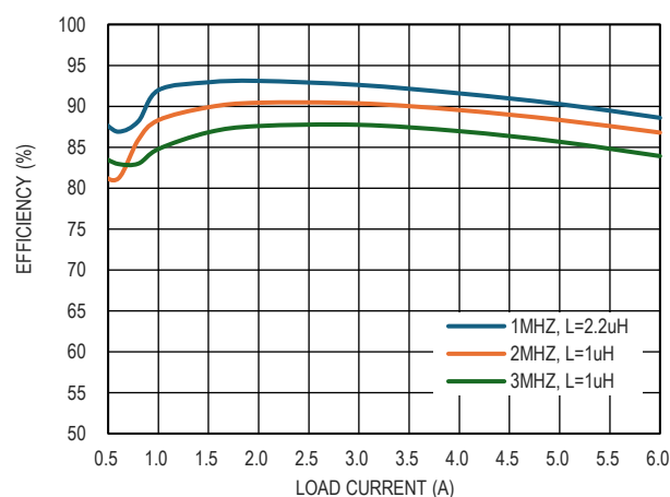
图 7. 效率曲线, V_{IN} = 12V , V_{OUT} = 3.3V
