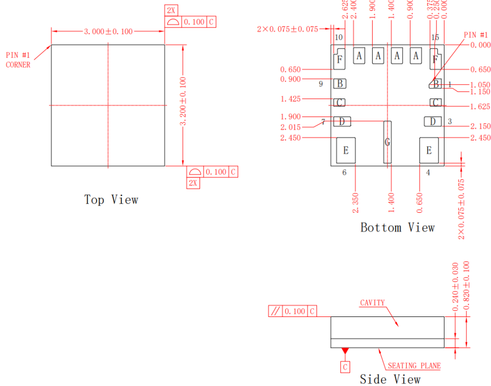
图 22.15 引脚 QFN
