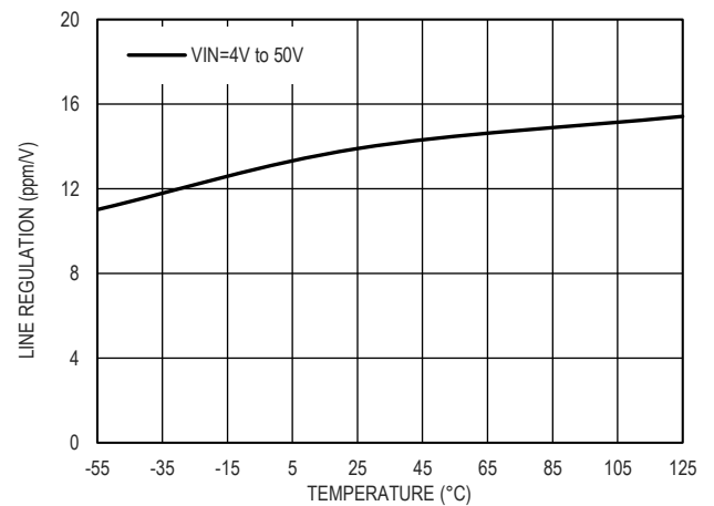
图 14. 输入调整率和温度的关系, V_{OUT}=3.0V
