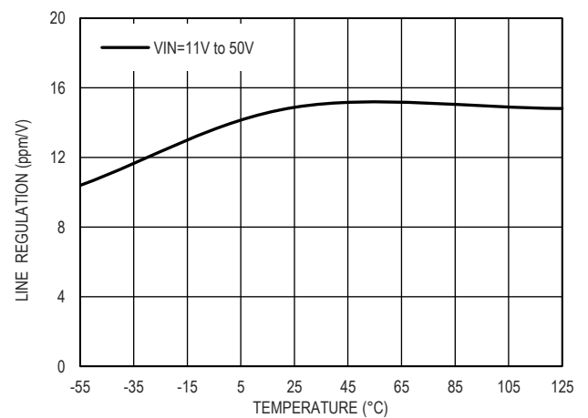
图 16. 输入调整率和温度的关系, V_{OUT}=10.0V
