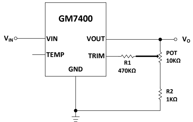
图 26. 输出电压微调电路
