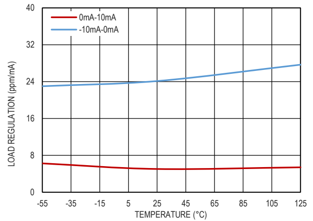
图 12. 负载调整率和温度的关系, V_{OUT}=10.0V
