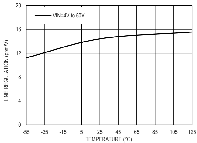
图 13. 输入调整率和温度的关系, V_{OUT}=2.5V
