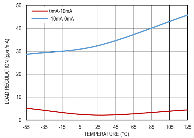
图 10. 负载调整率和温度的关系, V_{OUT}=3.0V
