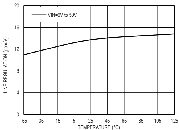
图 15. 输入调整率和温度的关系, V_{OUT}=5.0V
