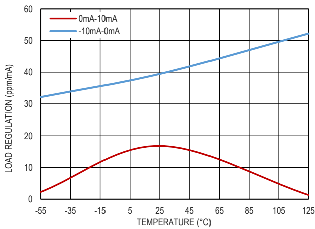
图 9. 负载调整率和温度的关系, V_{OUT}=2.5V
