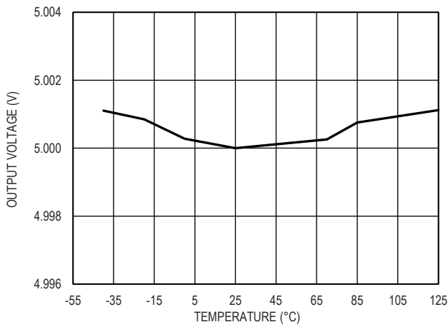
图 7. 5.0V 输出电压和温度的关系
