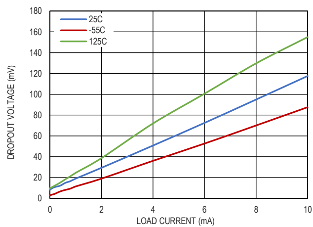
图 24.最小输入电压和输出电压的关系, V_{OUT}=10.0V
