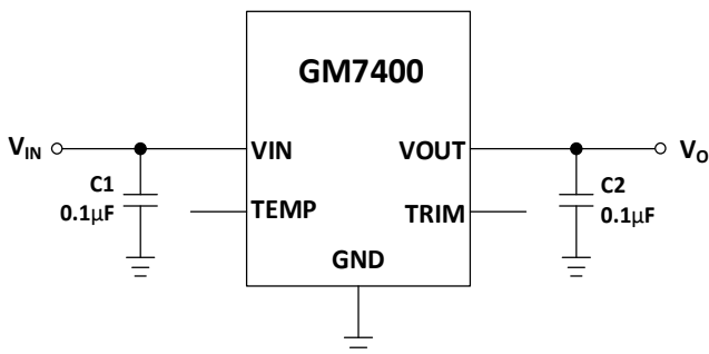
图 25. 有电容的应用电路
