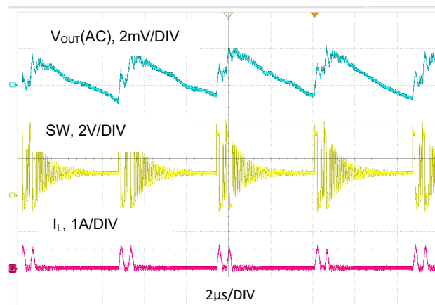
图 25. V_{OUT} = 1.2V , I_O = 100mA , PSM 模式
