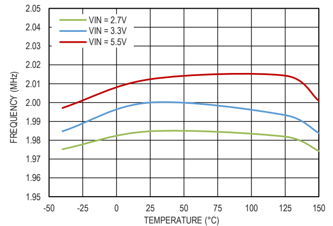
图 17. 频率和温度的关系, RT 接高
