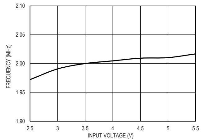
图 15. 频率和输入电压的关系, RT 接高
