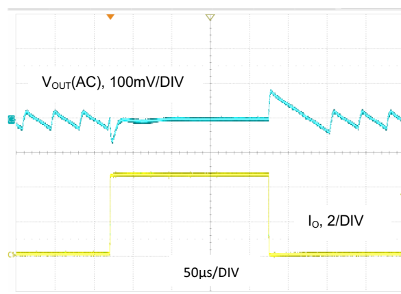
图 29. V_{OUT} = 1.2V , I_O = 0.1A 至 4.5A , 低功耗模式
