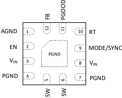
图 4 引脚配置
