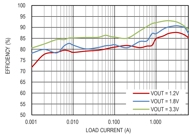
图 9. 效率曲线, V_{IN} = 5V , F_{SW} = 4MHz , 低功耗模式
