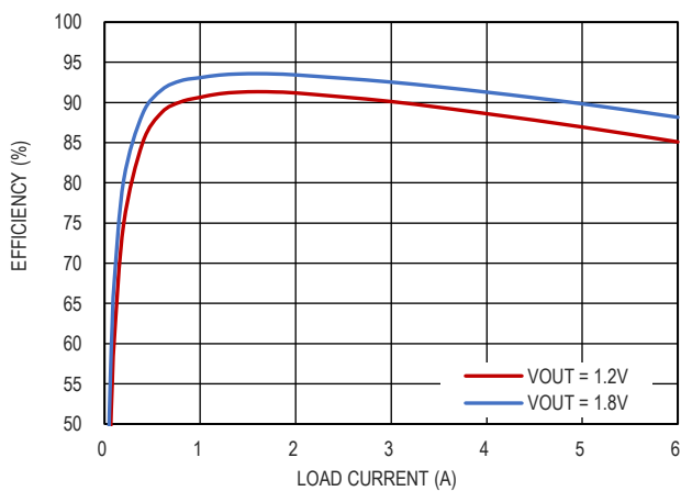
图 10. 效率曲线, V_{IN} = 3.3V , F_{SW} = 2MHz , FPWM
