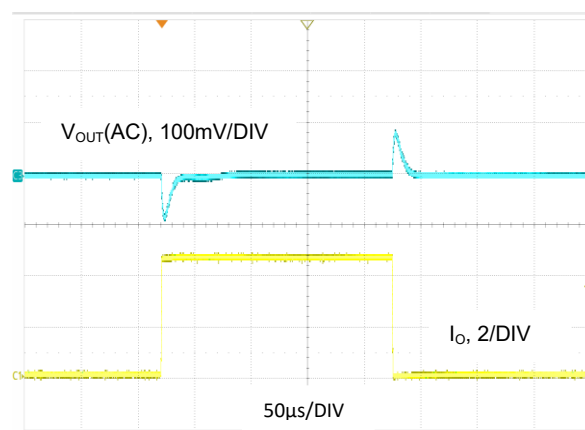
图 27. V_{OUT} = 1.2V , I_O = 0.1A 至 4.5A , FPWM 模式
