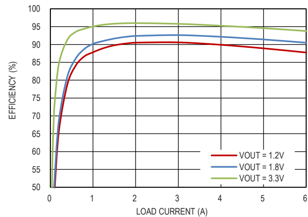
图 11. 效率曲线, V_{IN} = 5V , F_{SW} = 2MHz , FPWM
