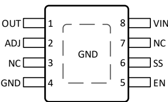
图 7. MSOP 引脚配置(顶视图)
