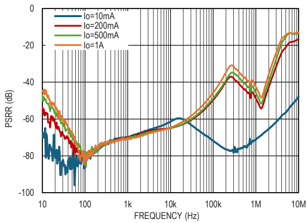
图 11. PSRR 和负载电流的关系, V_{OUT} = -15\text{V} , V_{IN} = -16\text{V}
