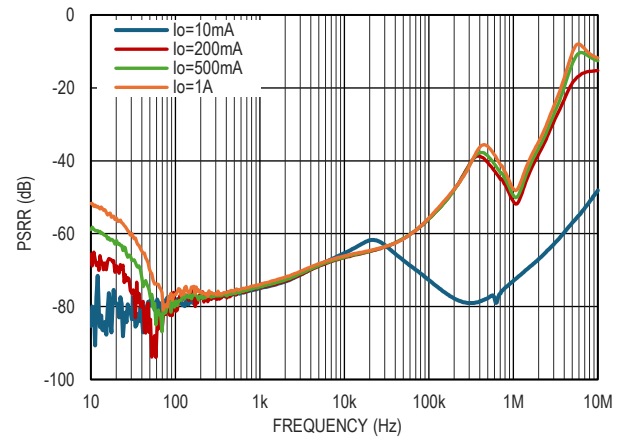
图 10. PSRR 和负载电流的关系, V_{OUT} = -5\text{V} , V_{IN} = -6\text{V}
