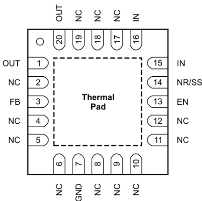
图 2. 5mm x 5mm QFN-20 引脚配置(顶视图)
