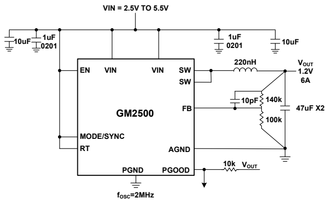
图 36. PGOOD 上拉至 V_{OUT}
