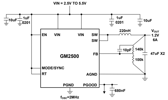
图 37. PGOOD 浮空
