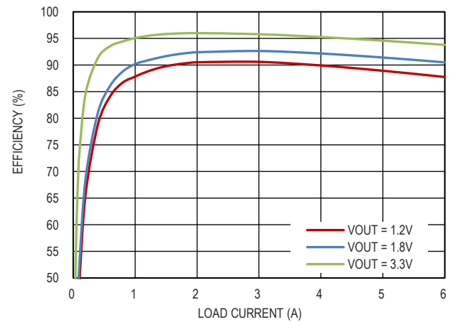
图 11. 效率曲线, V_{IN} = 5V , F_{SW} = 2MHz , FPWM
