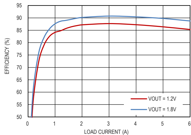
图 13. 效率曲线, V_{IN} = 5V , F_{SW} = 4MHz , FPWM
