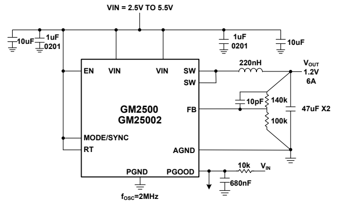
图 38. PGOOD 上拉至 V_{IN}
