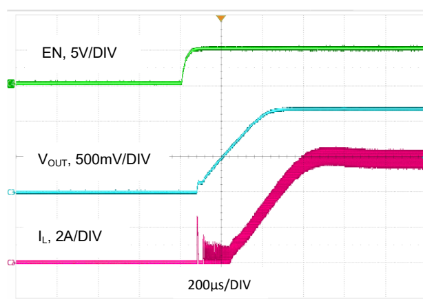
图 23. 启动波形, V_{OUT} = 1.2V , I_O = 6A
