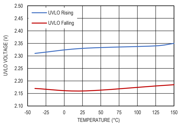
图 21. UVLO 阈值和温度的关系
