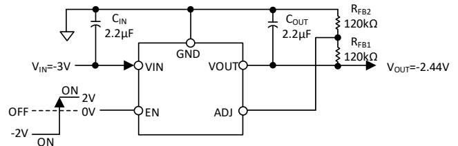
图 22. 设置可调输出电压
