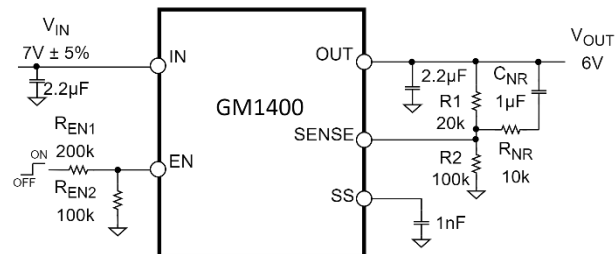
图 31. 噪声优化
