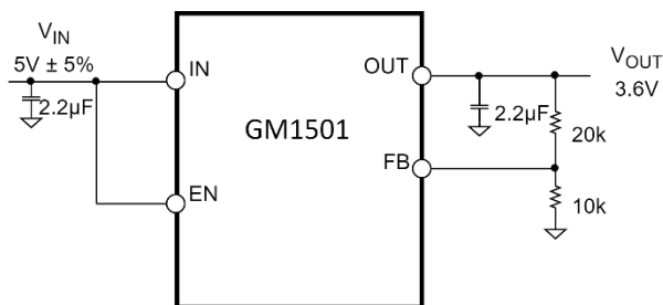
图 2. 可调输出至 3.6V
