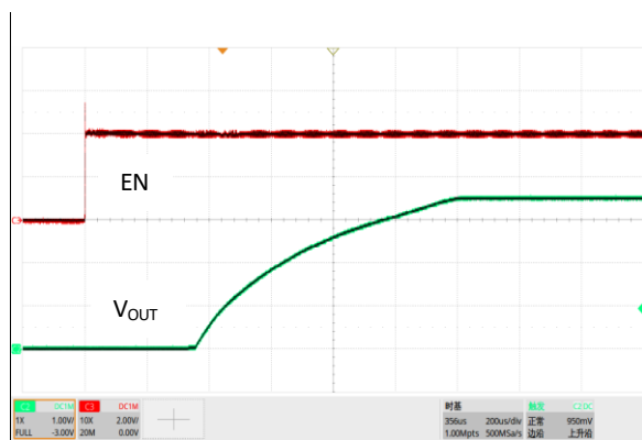
图 21. 软启动, V_{IN}=4.3V , V_{OUT}=3.6V , I_{OUT}=200mA
