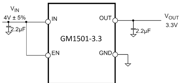
图 1. 固定输出 3.3V
