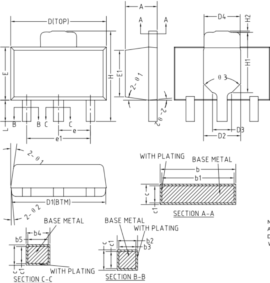
图 37. 3 引脚 SOT-89
