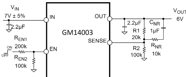
图 28. 噪声优化
