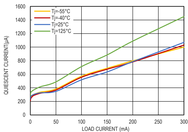
图 9. 静态电流和负载电流的关系, V_{IN} = 4.3\text{V}
