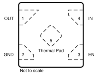
图 3.5 引脚 DFN-5 的引脚配置（固定输出，顶视图）
