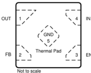
图 4.5 引脚 DFN-5 引脚配置（可调输出，顶视图）
