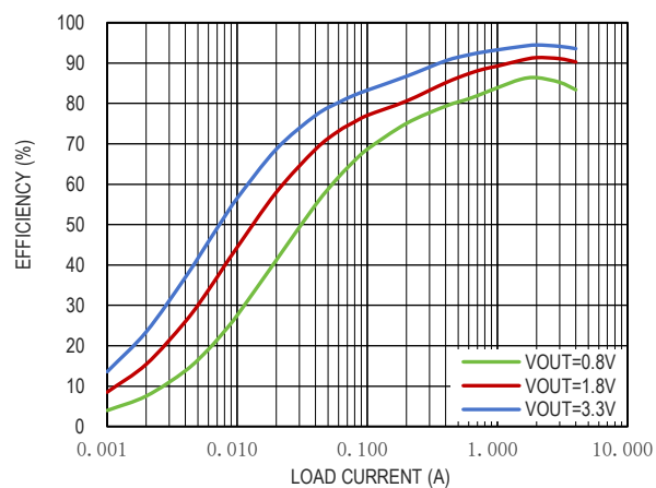
图 6. SKIP 模式效率曲线, V_{IN} = 5V
