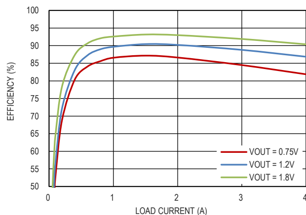
图 4. FPMW 模式效率曲线, V_{IN} = 3.3V
