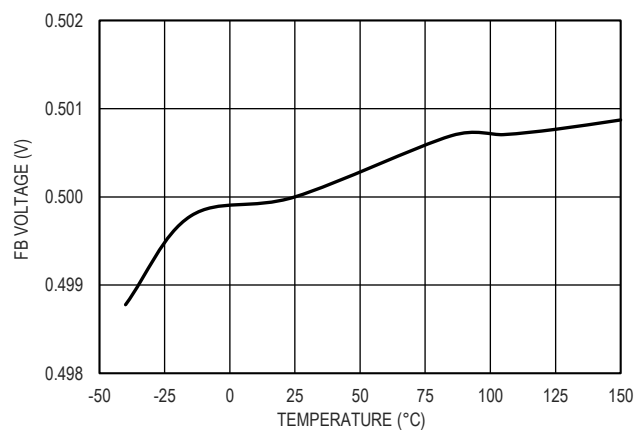
图 7. FB 引脚电压和温度的关系
