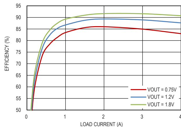
图 5. FPMW 模式效率曲线, V_{IN} = 5V
